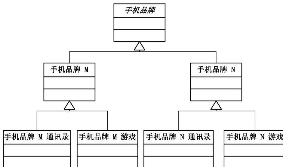
按软件分类实现结构图
