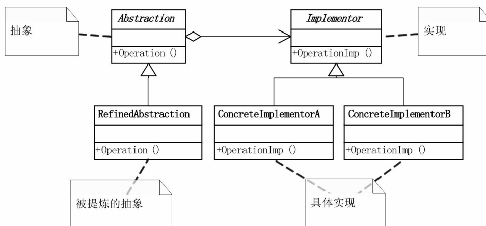
桥接模式 (Bridge) 结构图
