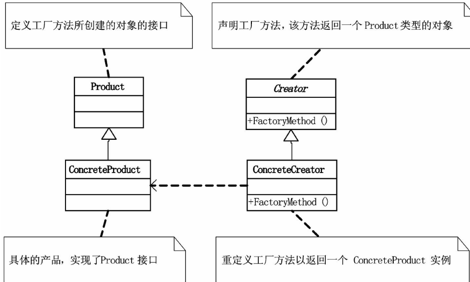
工厂方法模式 (Factory Method) 结构图
