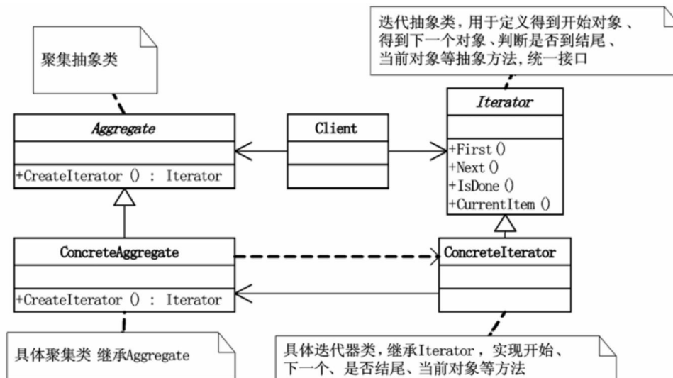
23号选手 迭代器 (Iterator)
