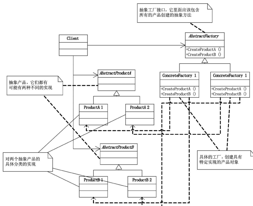
抽象工厂模式（ Abstract Factory ）结构图
