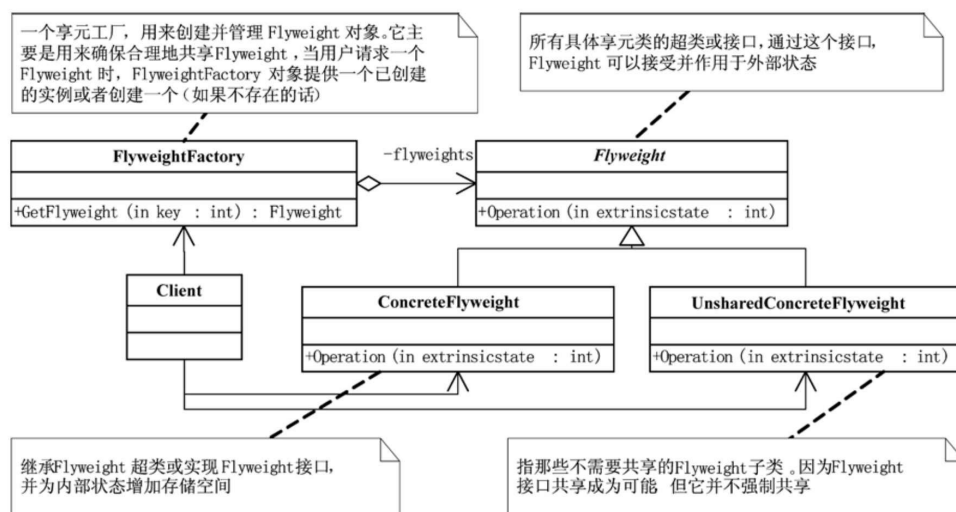
享元模式（flyweight）结构图
