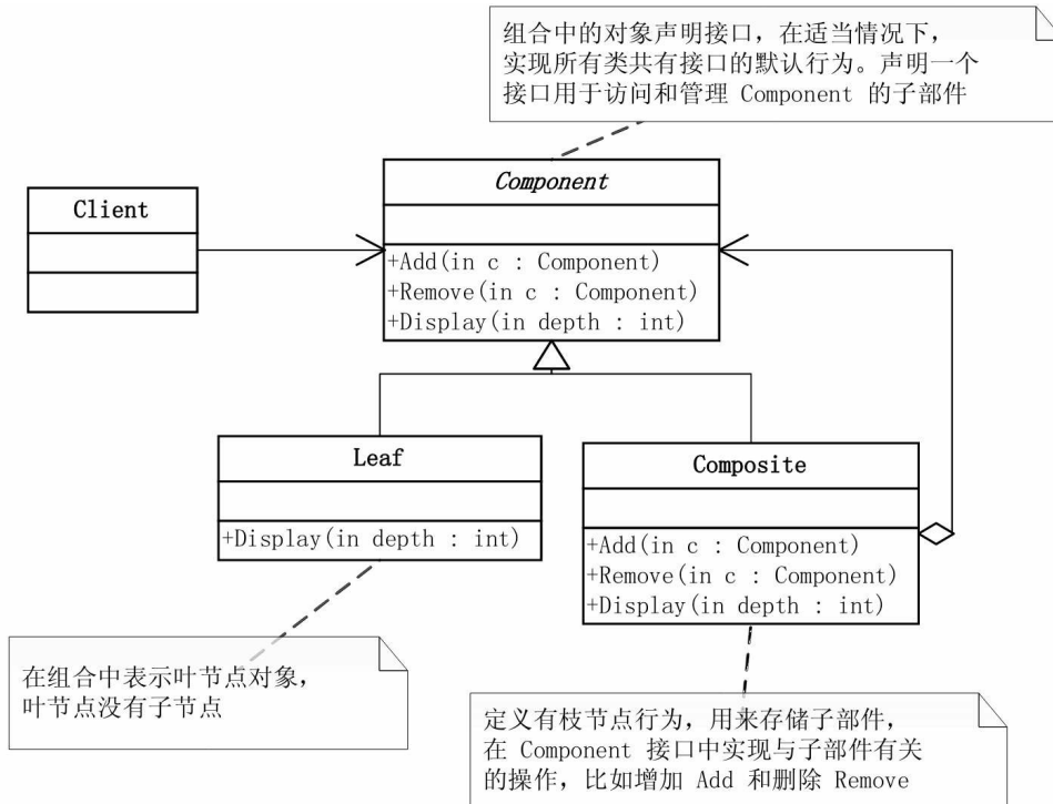
组合模式 (Composite) 结构图
