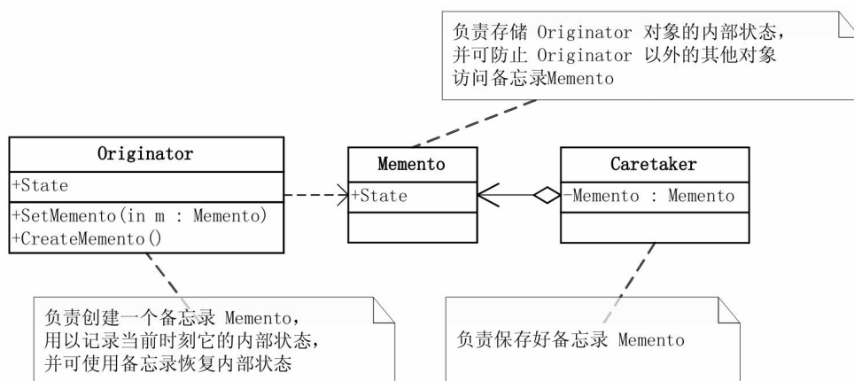
备忘录模式 (Memento) 结构图
