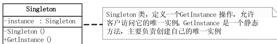
单例模式 (Singleton) 结构图
