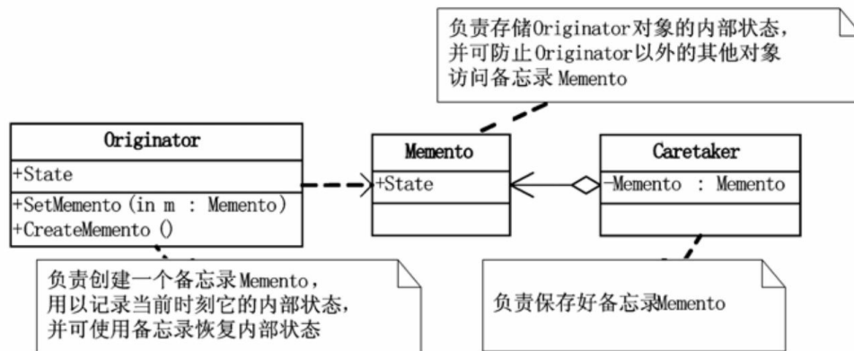
22号选手 备忘录 (Memento)
