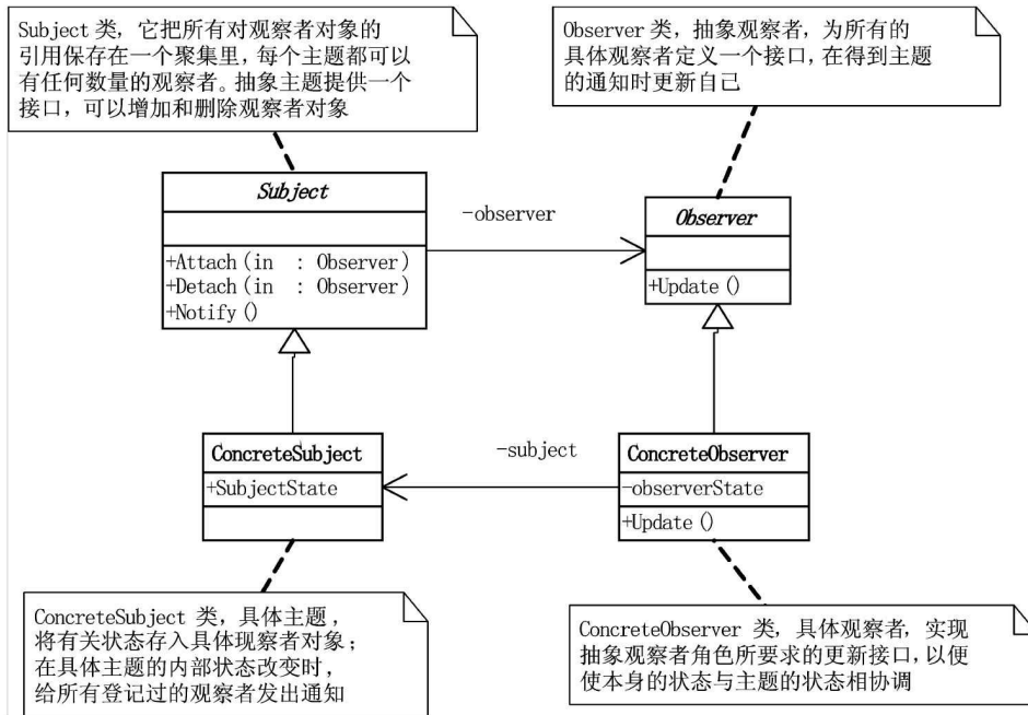
观察者模式（Observer）结构图
