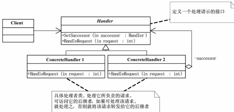
职责链模式 (Chain of Responsibility) 结构图
