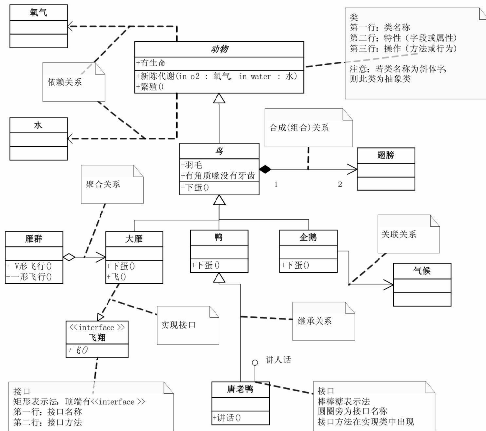
UML类图图示样例
