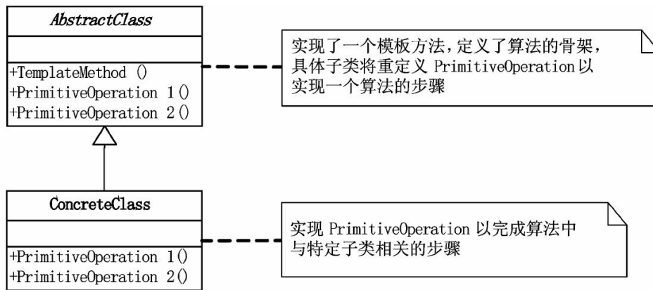
模板方法模式 (TemplateMethod) 结构图
