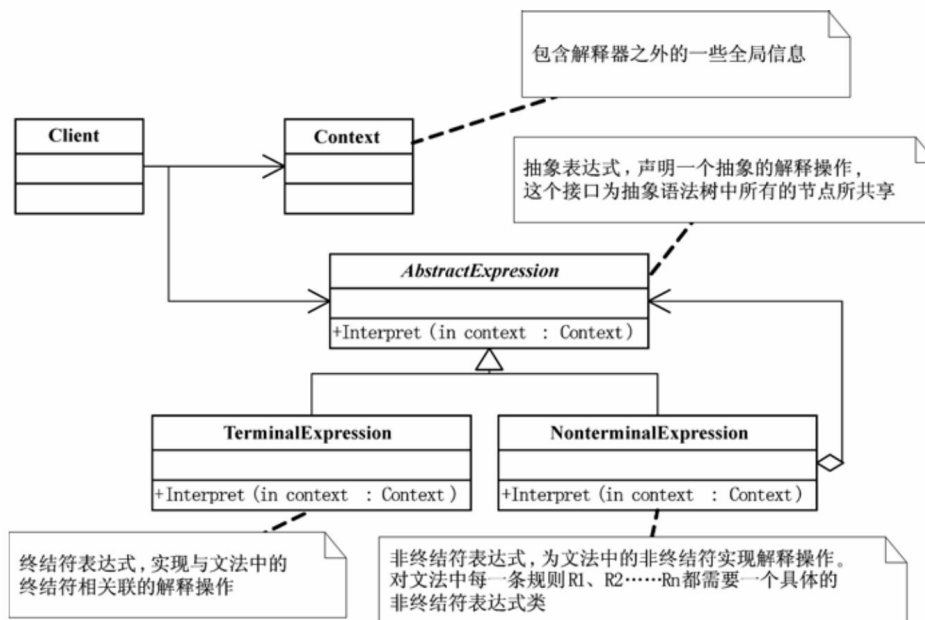
解释器模式 (interpreter) 结构图
