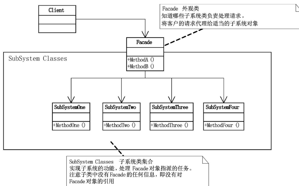
外观模式 (Facade) 结构图
