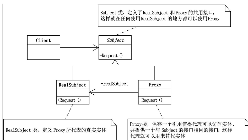
代理模式 ( Proxy ) 结构图
