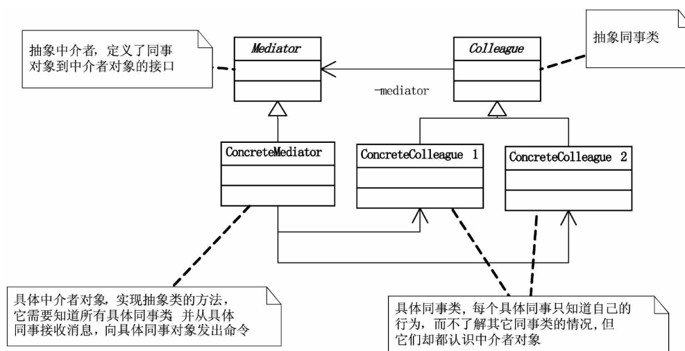
中介者模式 (Mediator) 结构图
