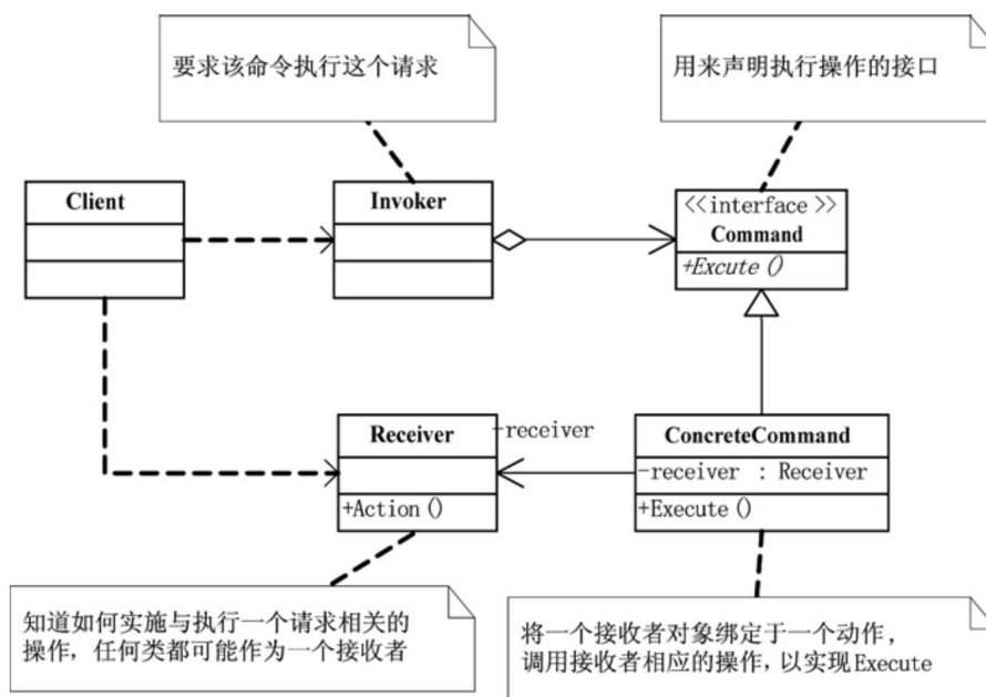
命令模式 (Command) 结构图
