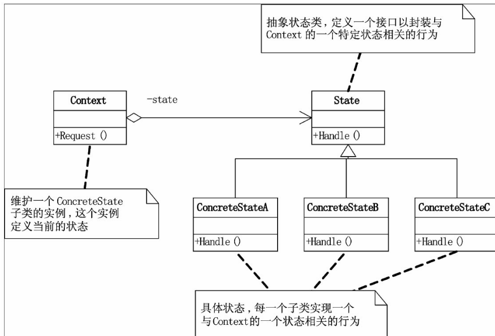
状态模式 (State) 结构图
