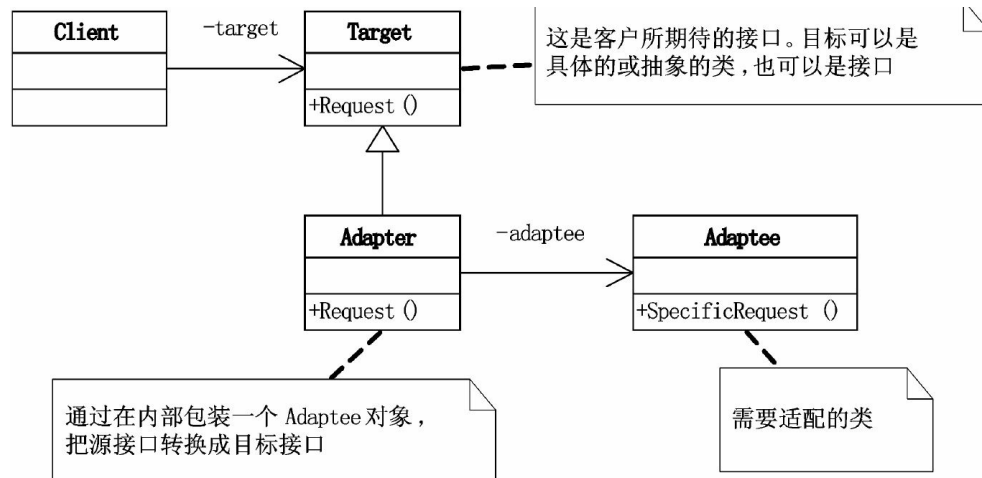
适配器模式 (Adapter) 结构图
