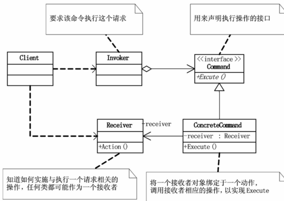
15号选手 命令 (Command)
