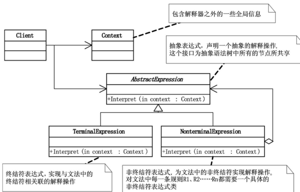
18号选手 解释器 (interpreter)
