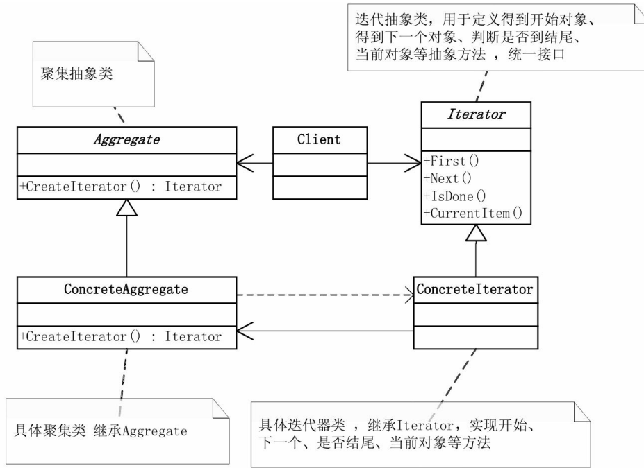
迭代器模式 (Iterator) 结构图
