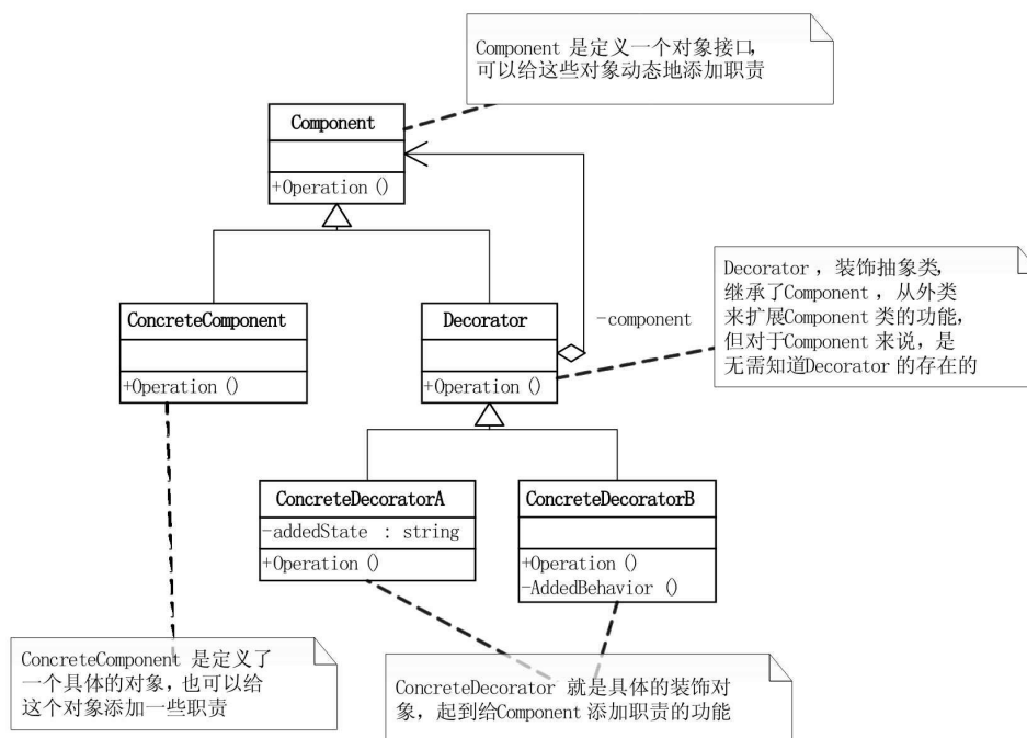
装饰模式 (Decorator) 结构图
