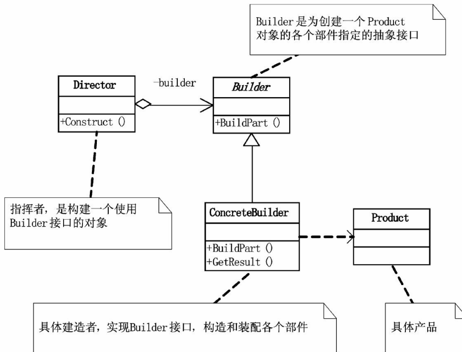
建造者模式 (Builder) 结构图
