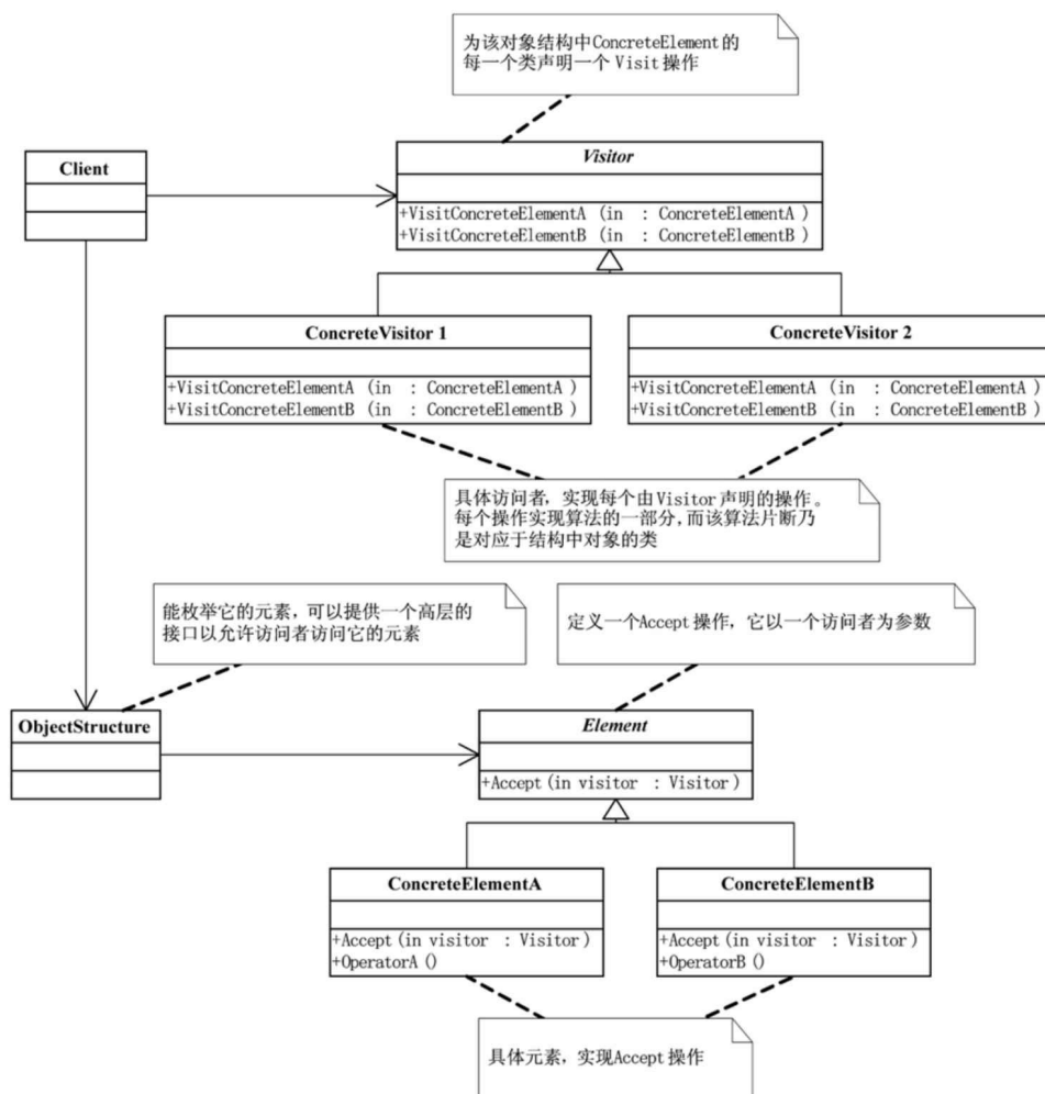
访问者模式（Visitor）结构图
