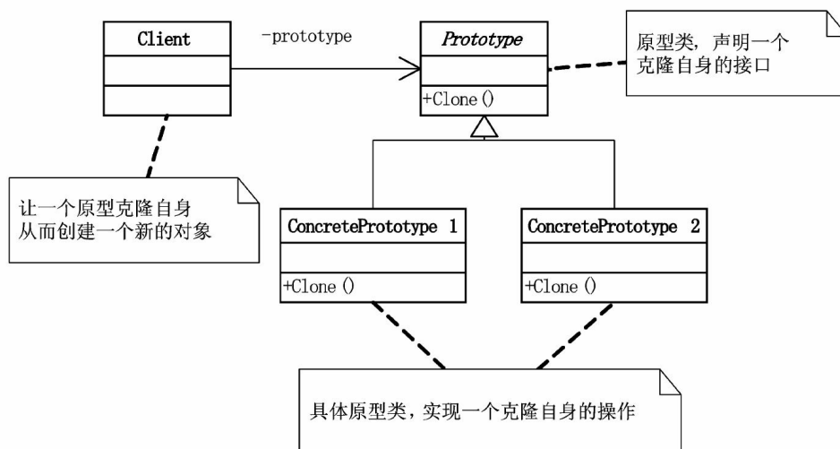
原型模式 (Prototype) 结构图
