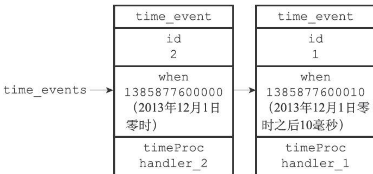
图12-9 用链表连接起来的两个时间事件
