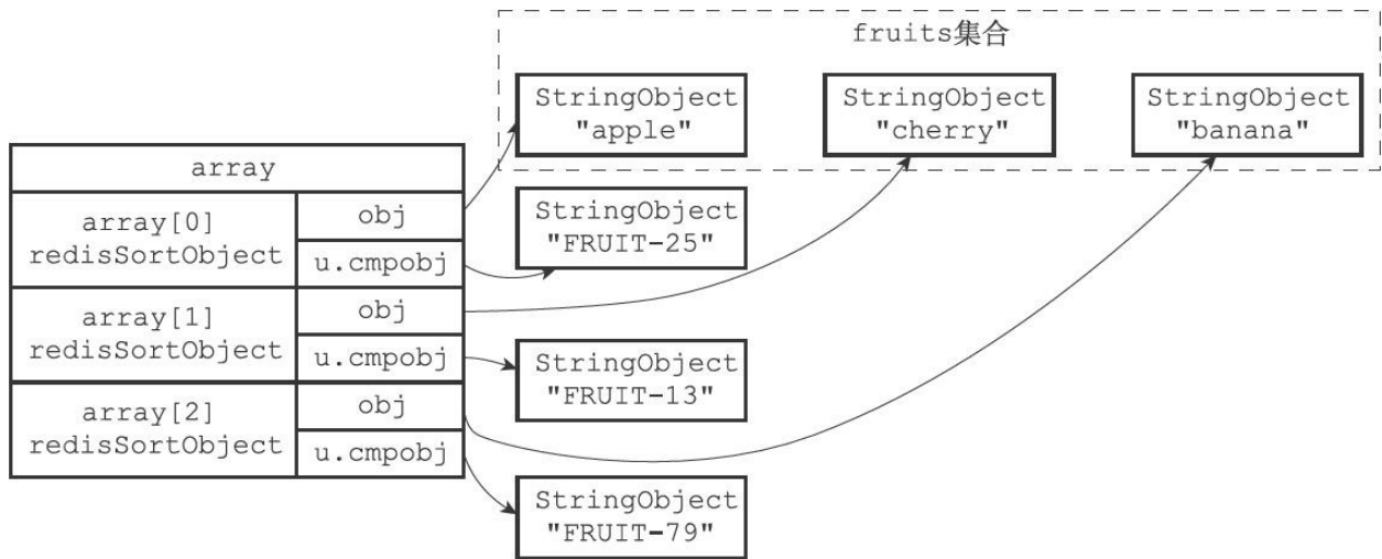
图21-13 将u.cmpobj指针指向权重键
