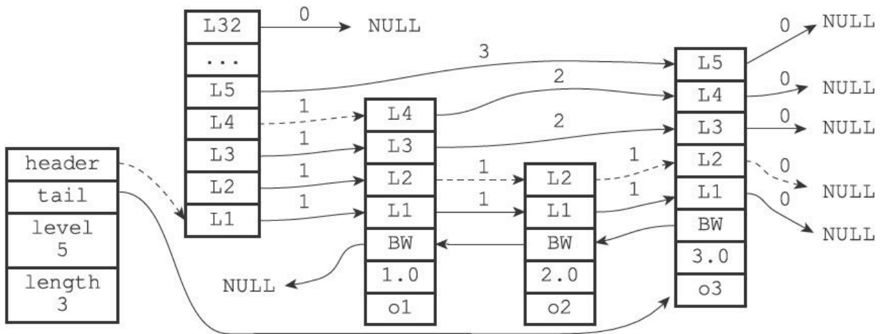
图5-3 遍历整个跳跃表
