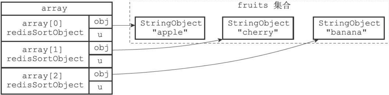
图21-5 将obj指针指向集合的各个元素
