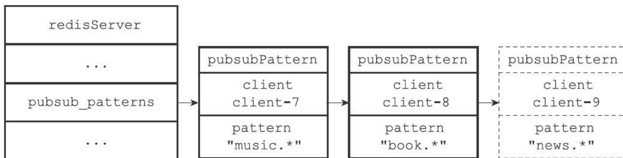
图18-13 执行PSUBSCRIBE命令之后的pubsub_patterns链表
