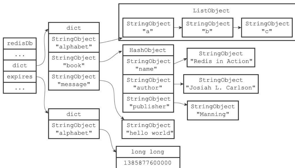
图9-14 执行PERSIST之后的数据库
