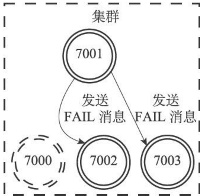
图17-43 节点7001向集群广播FAIL消息
