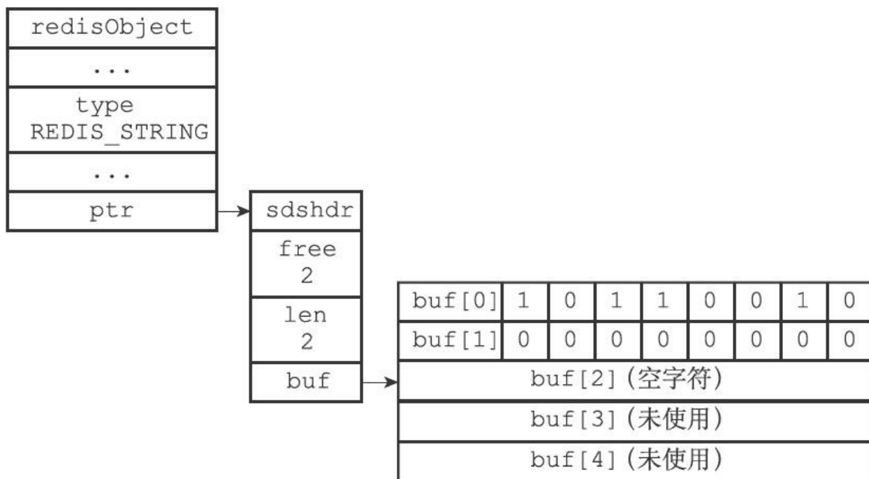
图22-8 扩展空间之后的位数组
