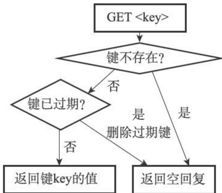
图9-16 GET命令的执行过程
