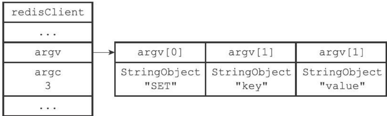
图13-5 argv属性和argc属性示例
