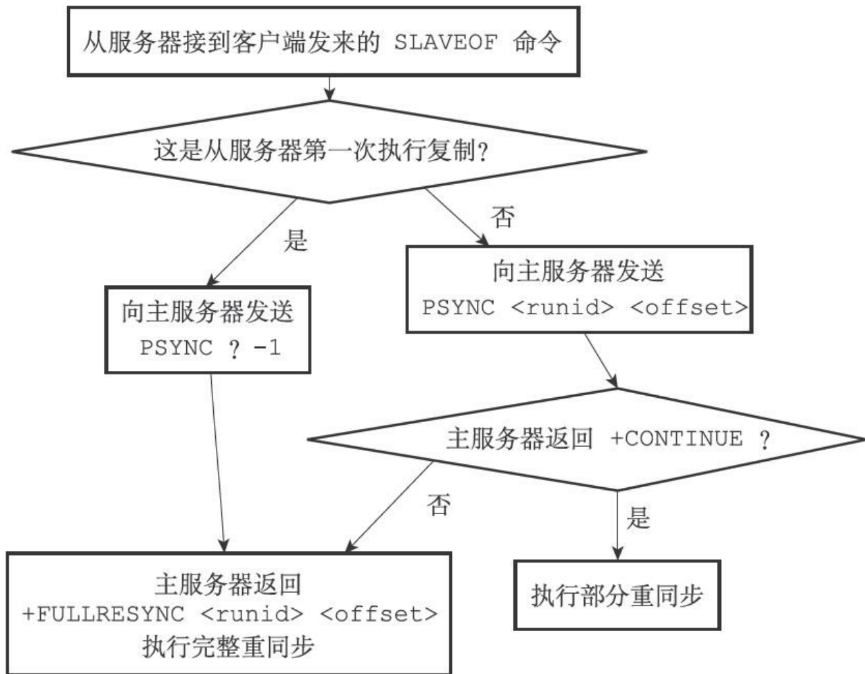
图15-12 PSYNC执行完整重同步和部分重同步时可能遇到的情况
