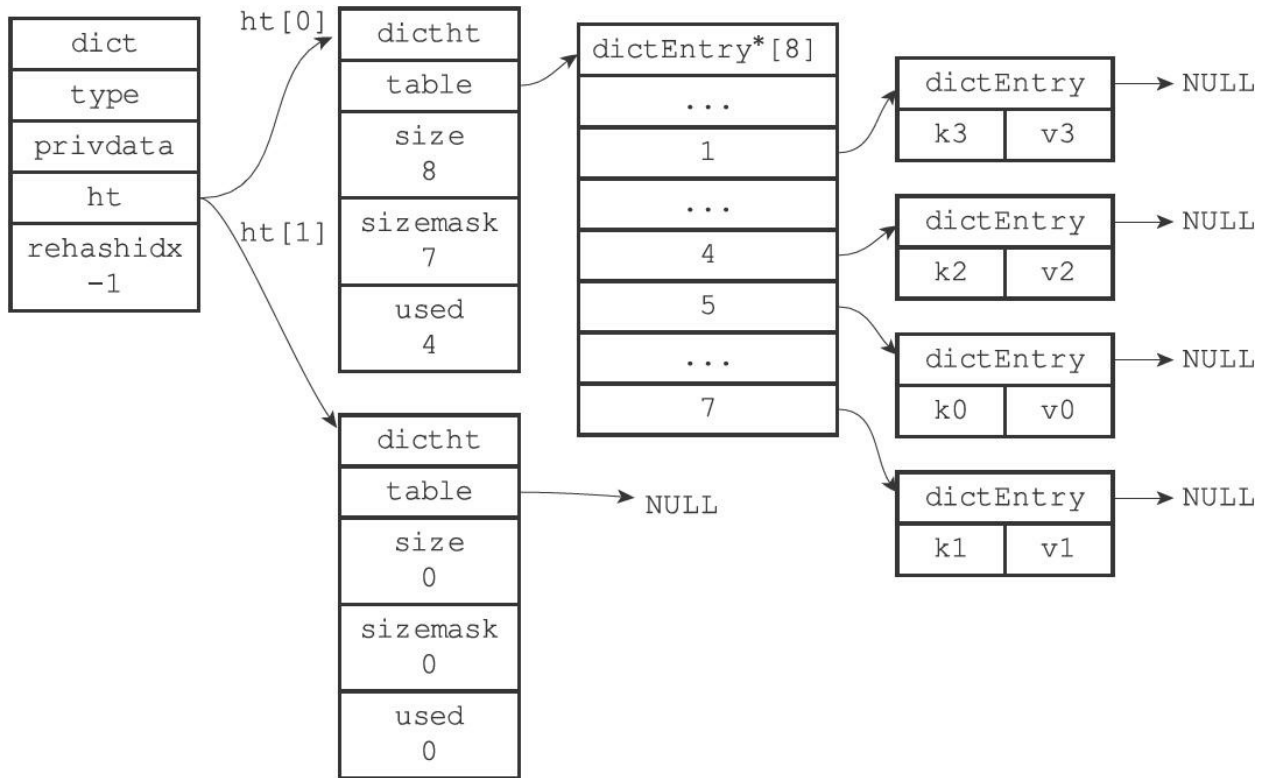
图4-11 完成rehash之后的字典
