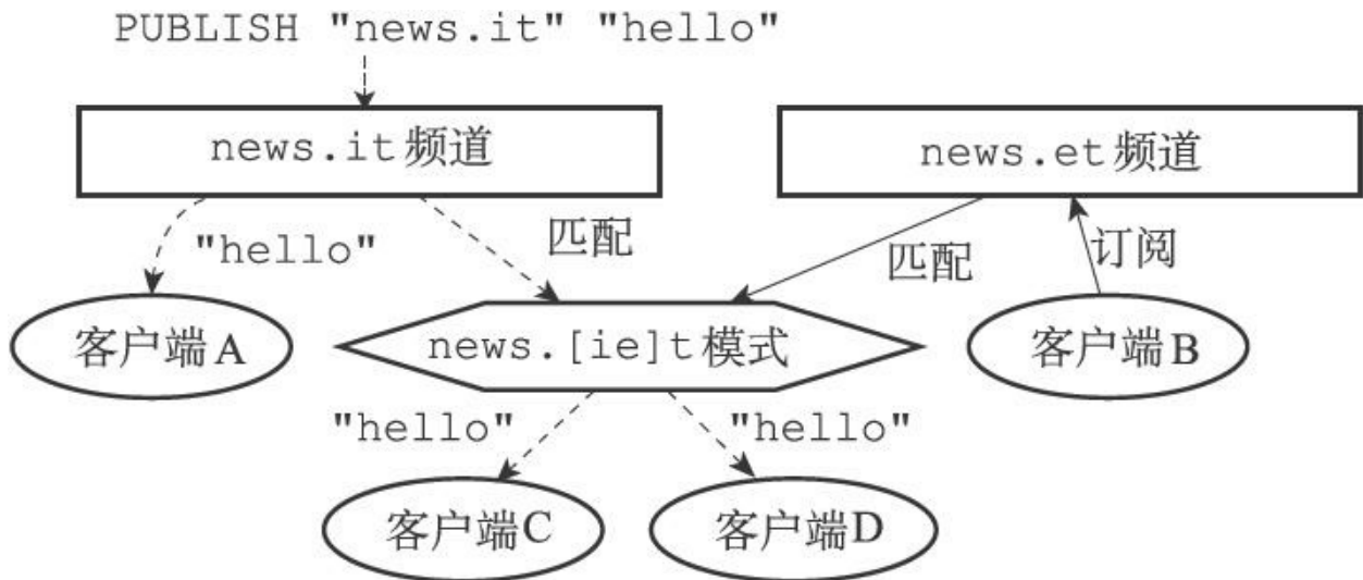
图18-4 将消息发送给频道的订阅者和匹配模式的订阅者 (1)
