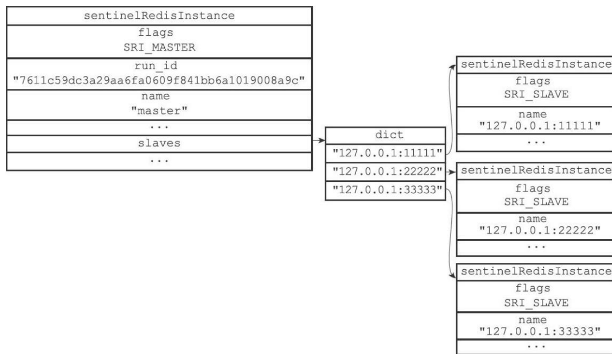
图16-10 主服务器和它的三个从服务器
