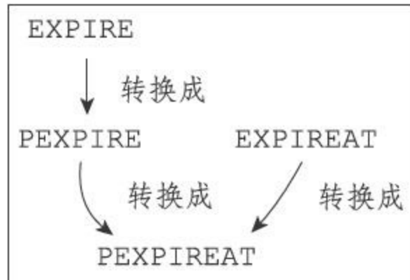
图9-11 设置生存时间和设置过期时间的命令之间的转换
