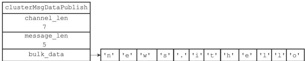
图17-46 clusterMsgDataPublish结构示例
