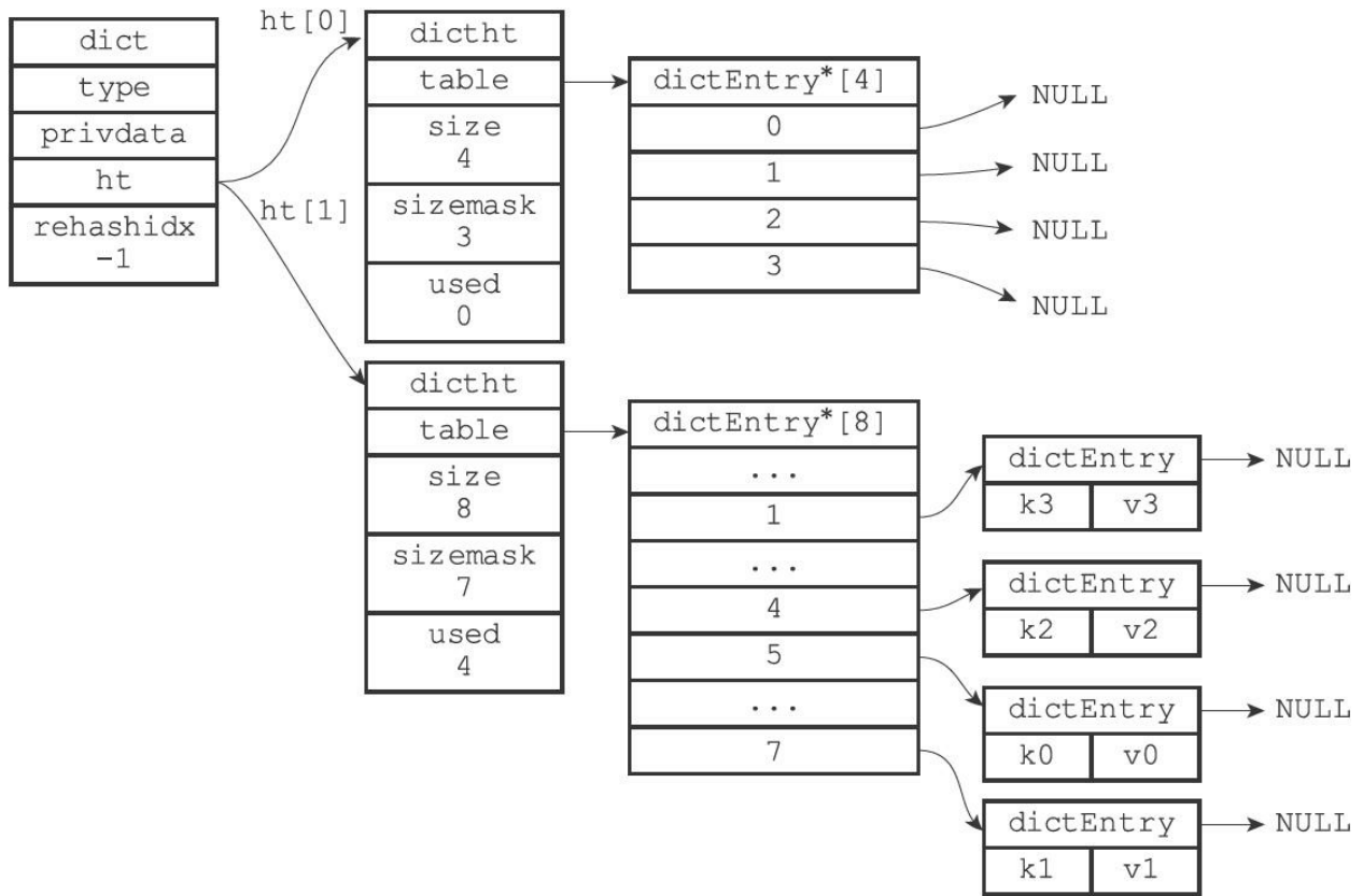
图4-10 ht[0] 的所有键值对都已经被迁移到 ht[1]
