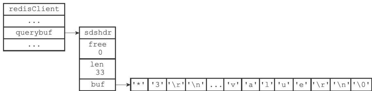
图13-4 querybuf属性示例
