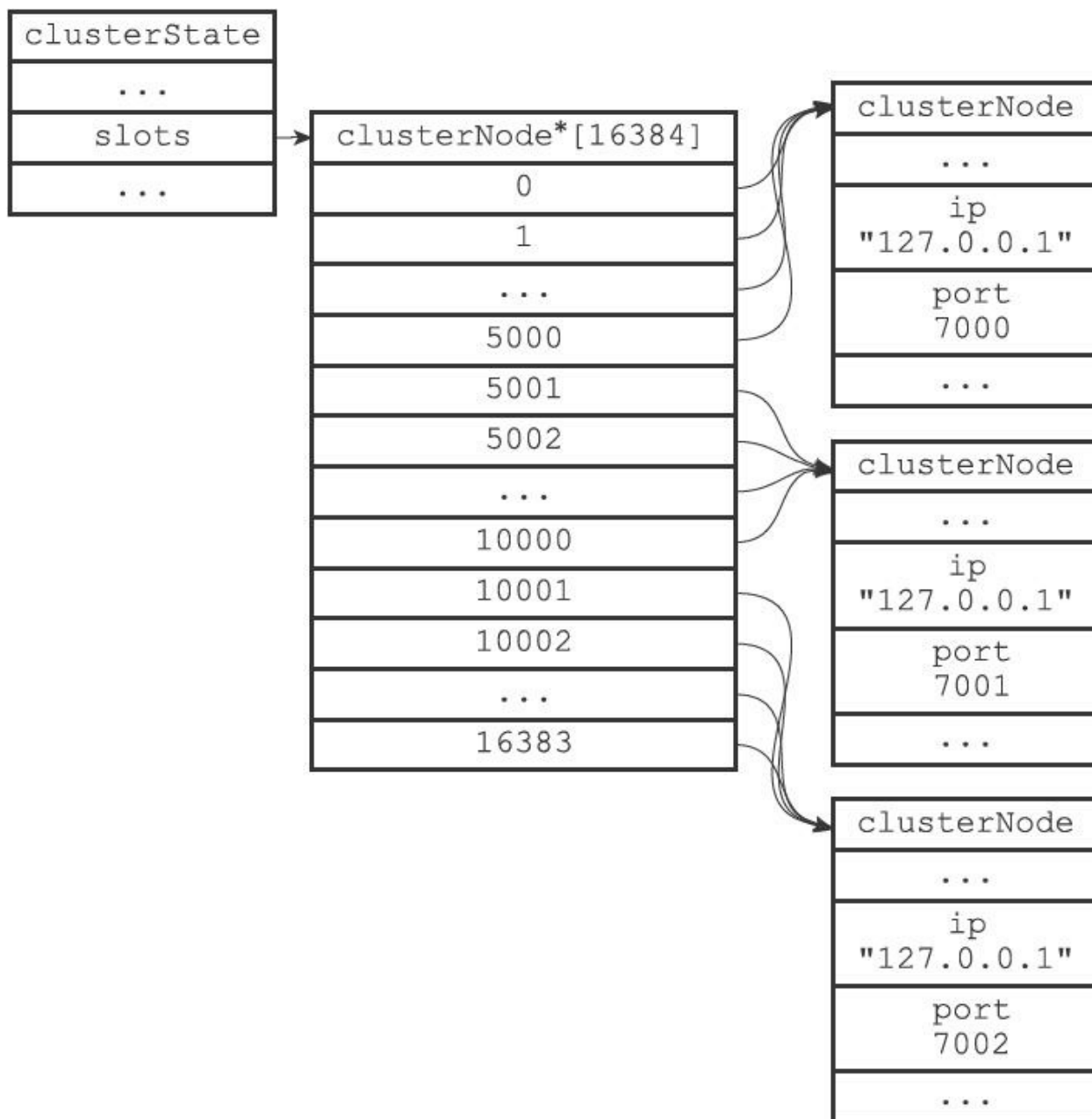
图17-14 clusterState结构的slots数组
