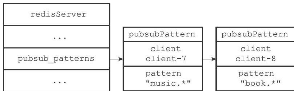
图18-12 执行PSUBSCRIBE命令之前的pubsub_patterns链表
