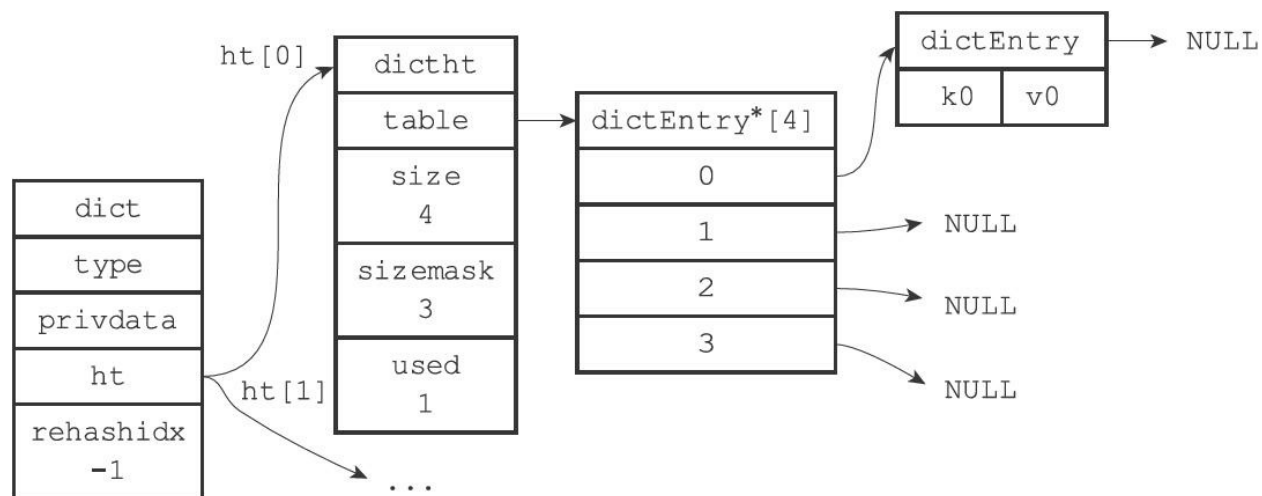
图4-5 添加键值对 k_0 和 v_0 之后的字典
