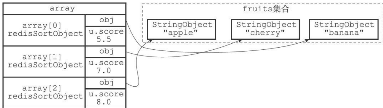
图21-11 根据u.score属性进行排序之后的数组
