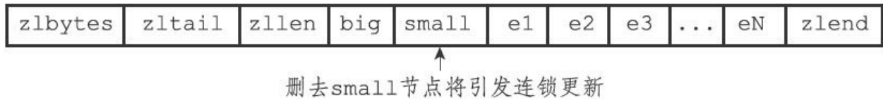
图7-14 另一种引起连锁更新的情况
