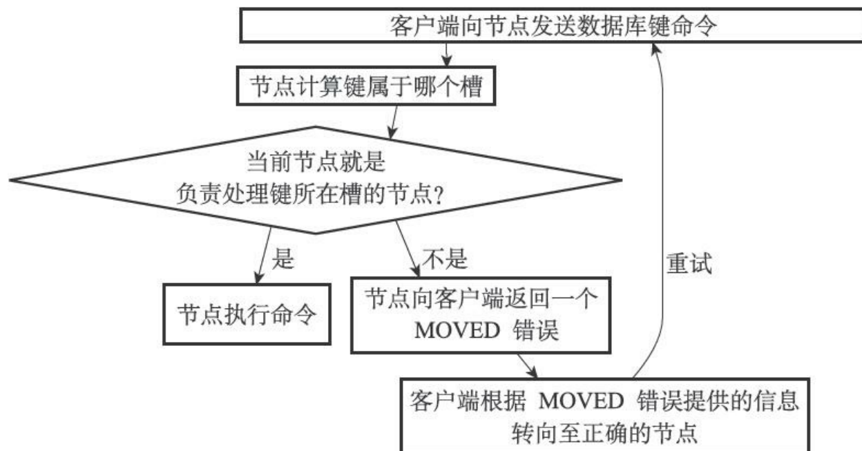
图17-18 判断客户端是否需要转向的流程
