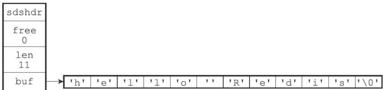
图2-19 一个保存着文本数据的SDS
