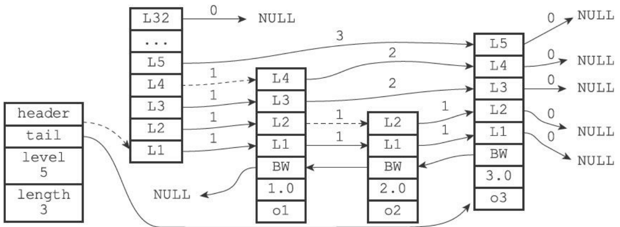
图5-5 另一个计算节点排位的例子
