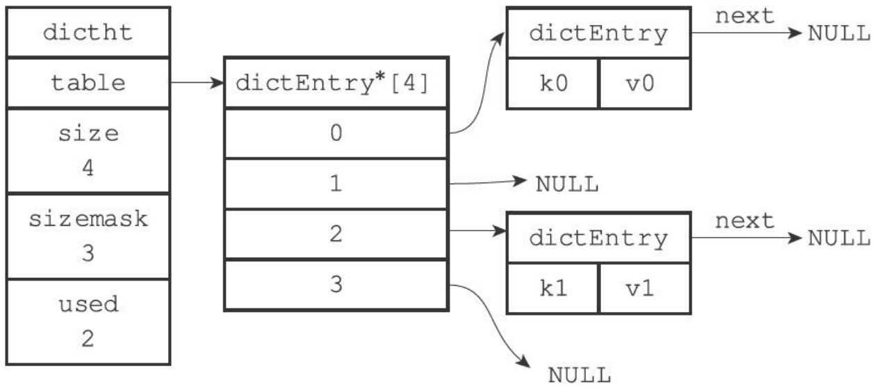
图4-6 一个包含两个键值对的哈希表
