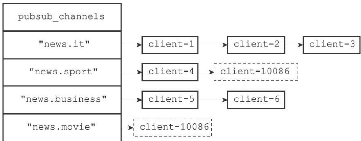
图18-7 执行SUBSCRIBE之后的pubsub_channels字典
