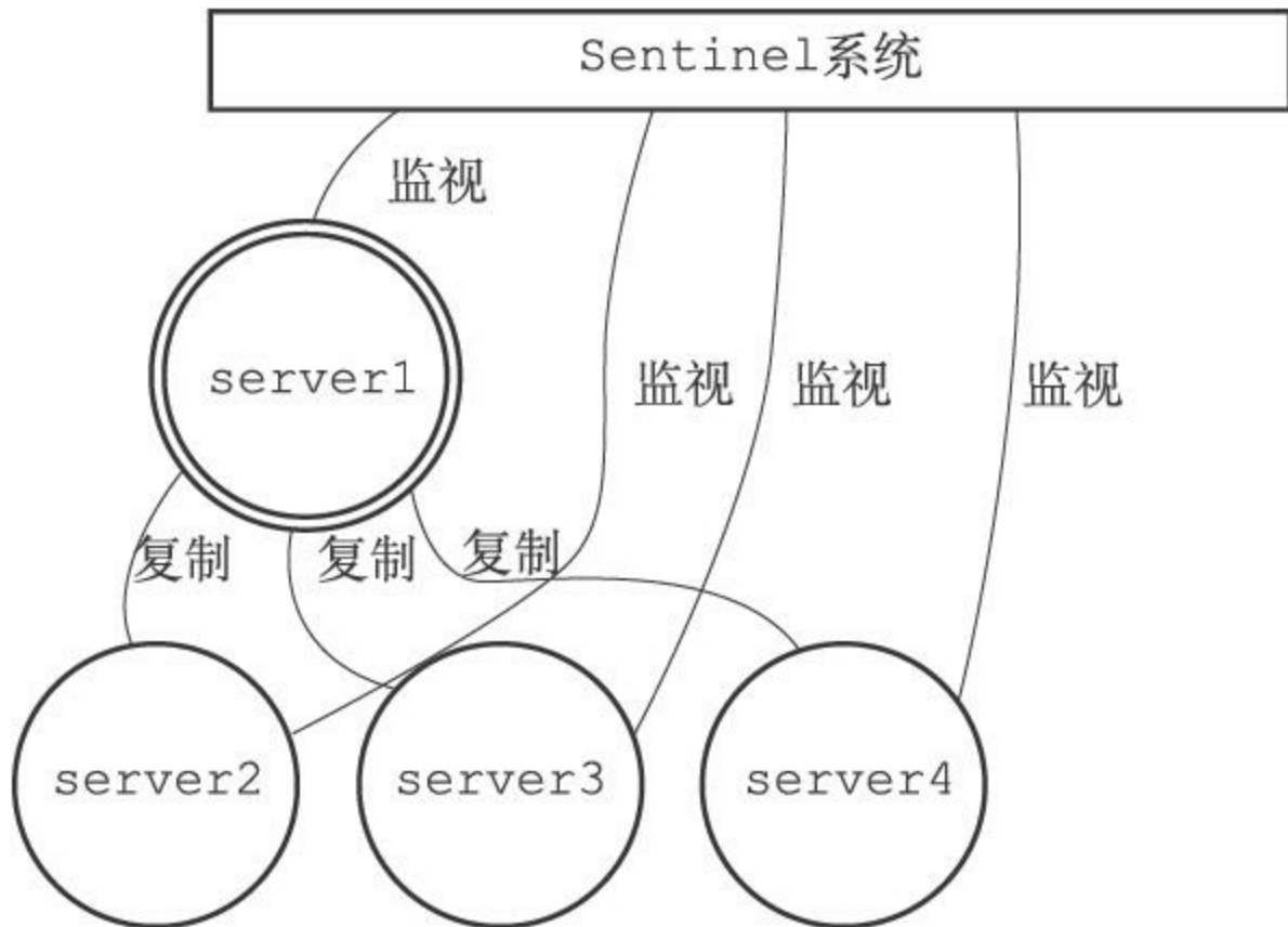
图16-1 服务器与Sentinel系统
