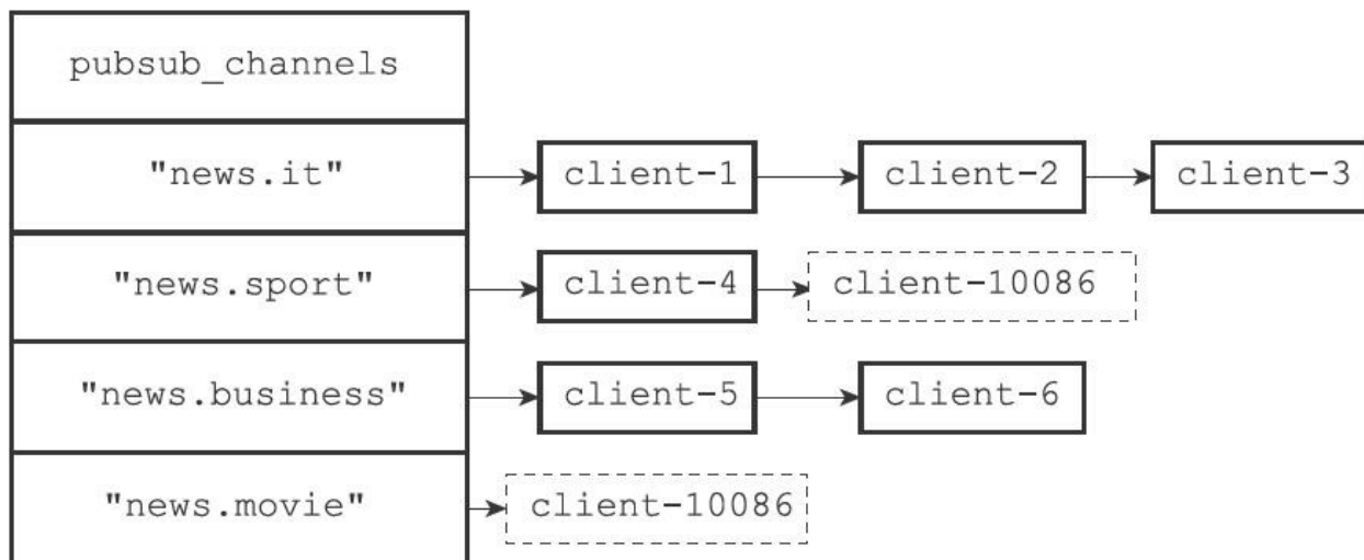
图18-8 执行UNSUBSCRIBE之前的pubsub_channels字典
