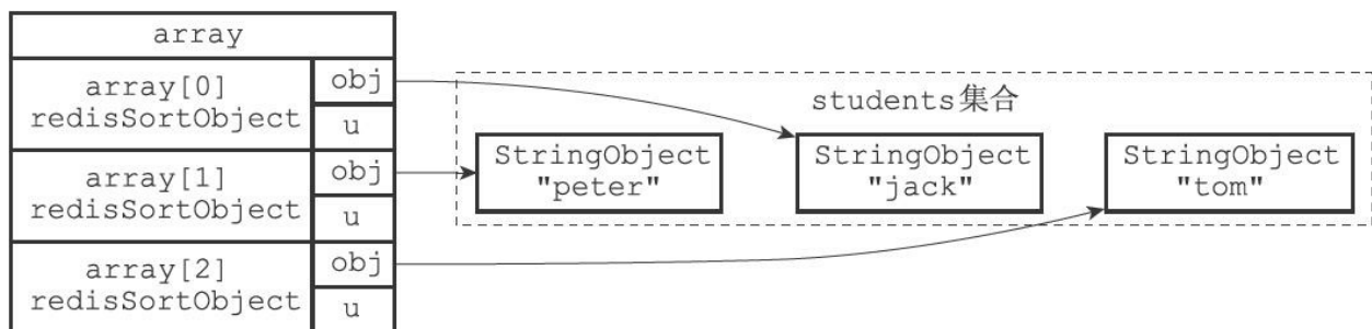
图21-19 排序之后的数组
