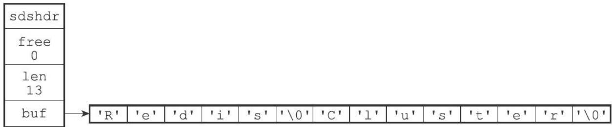
图2-18 保存了特殊数据格式的SDS
