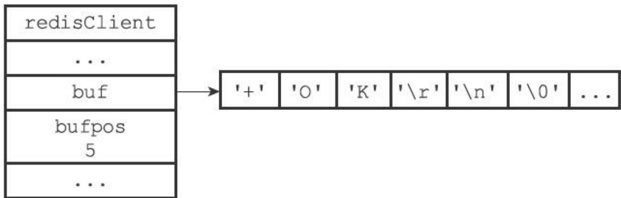
图14-7 保存了命令回复的客户端状态
