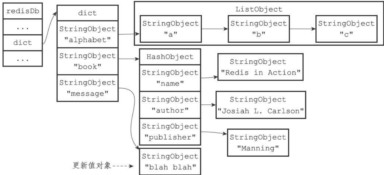
图9-7 使用SET命令更新message键
