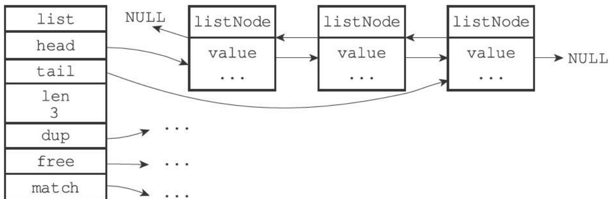
图3-2 由list结构和listNode结构组成的链表
