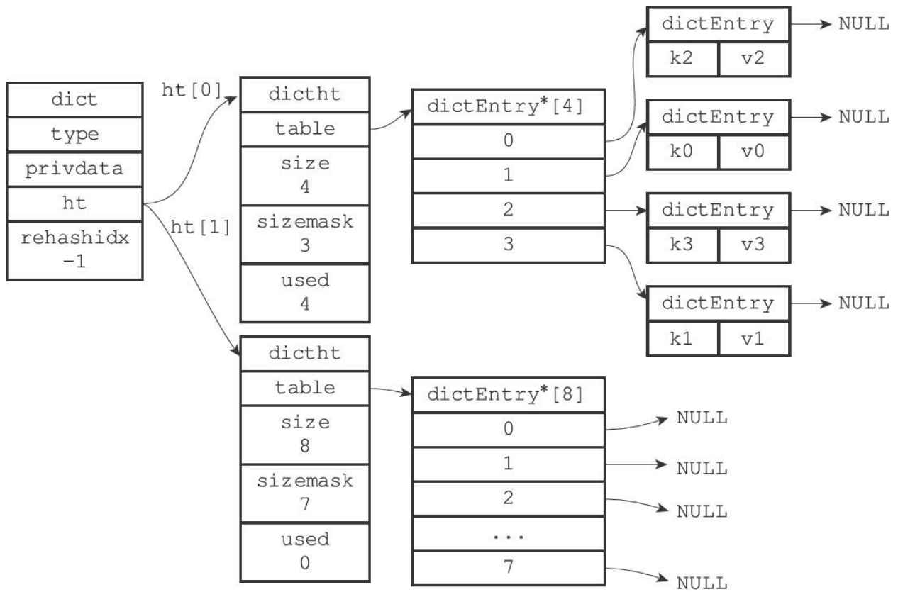
图4-9 为字典的ht[1]哈希表分配空间
