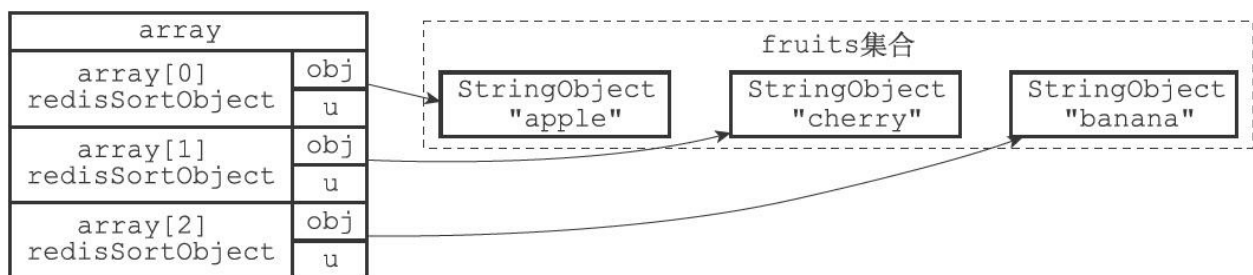
图21-9 将obj指针指向集合的各个元素
