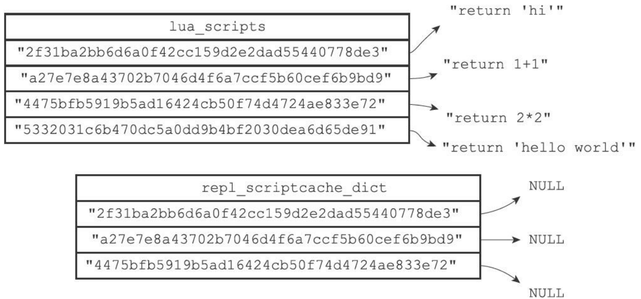
图20-13 执行EVALSHA命令之前的lua_scripts字典和repl_scriptcache_dict字典
