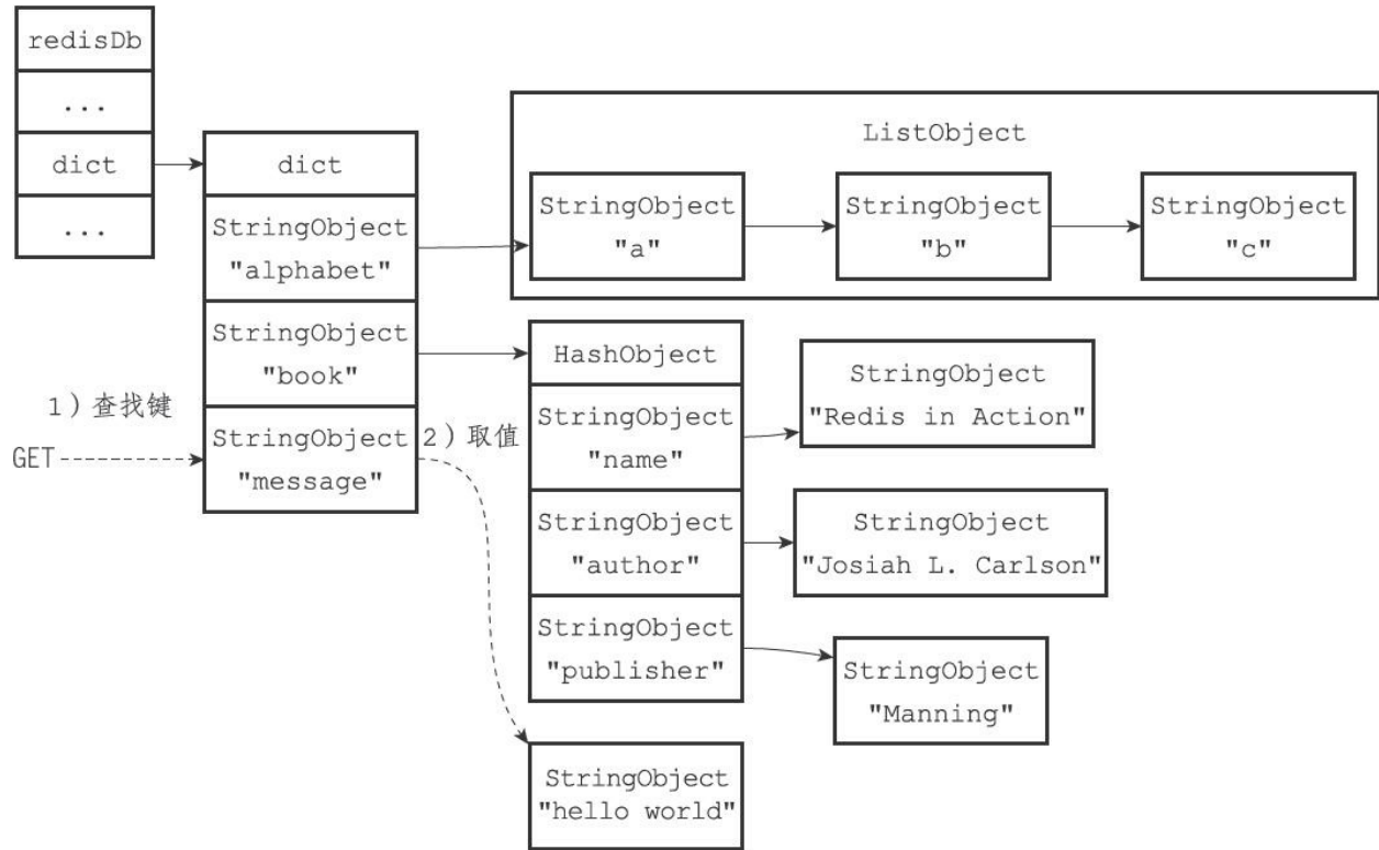
图9-9 使用GET命令取值的过程
