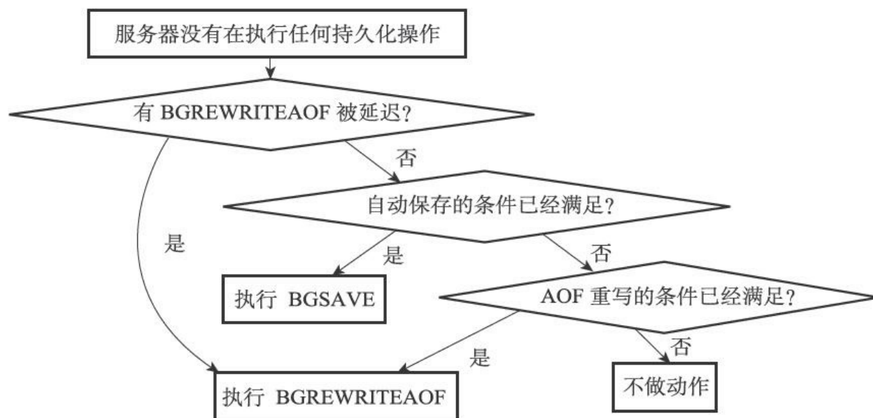
图14-9 判断是否需要执行持久化操作
