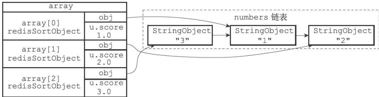
图21-7 执行升序排序的数组
