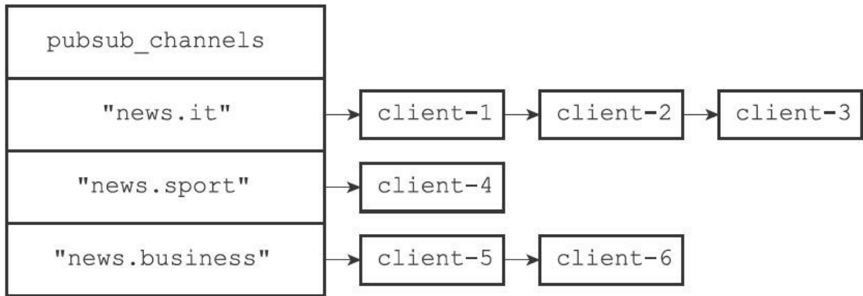
图18-9 执行UNSUBSCRIBE之后的pubsub_channels字典
