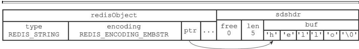
图8-4 embstr编码的字符串对象
