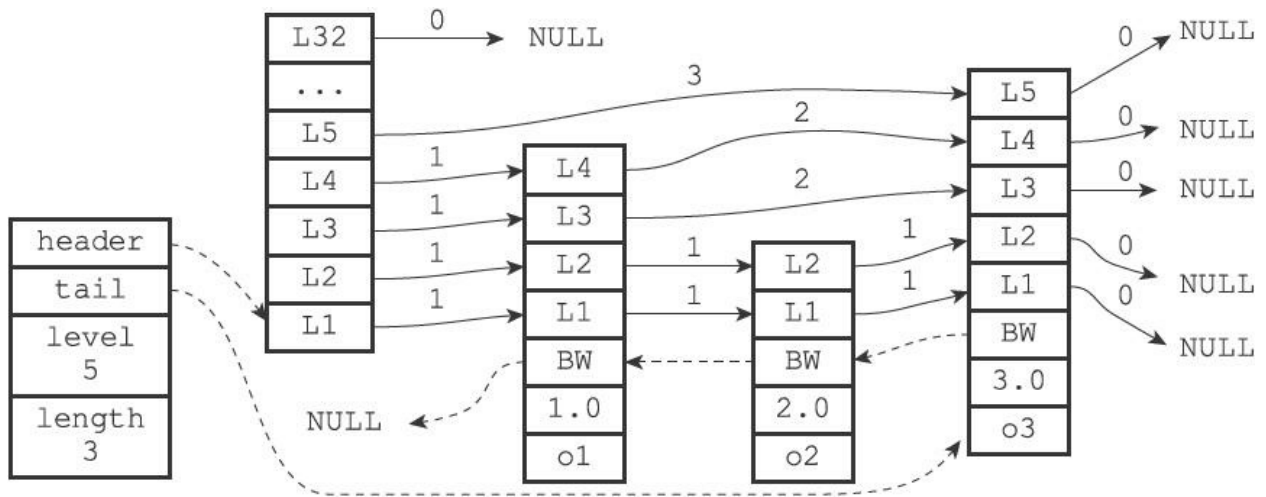
图5-6 从表尾向表头方向遍历跳跃表
