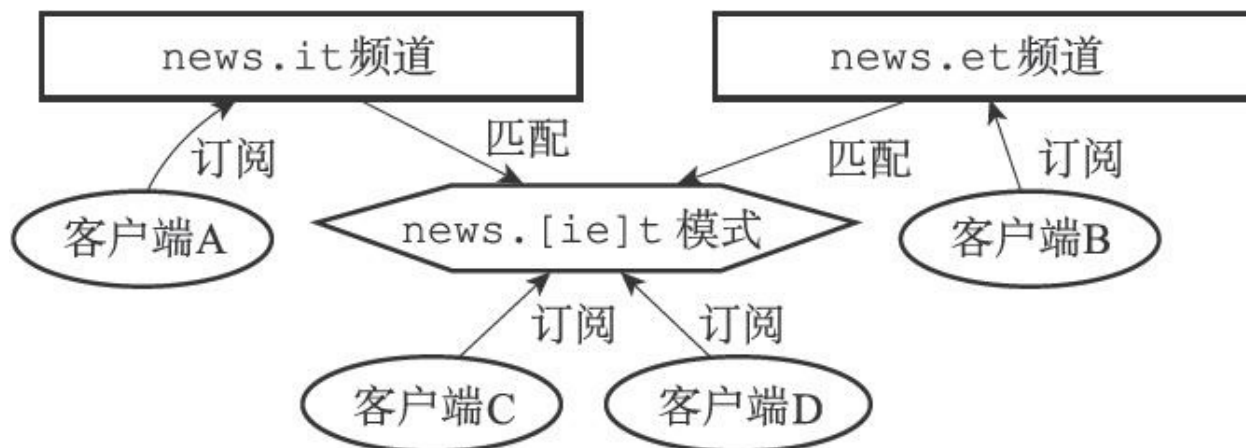
图18-3 频道和模式的订阅状态
