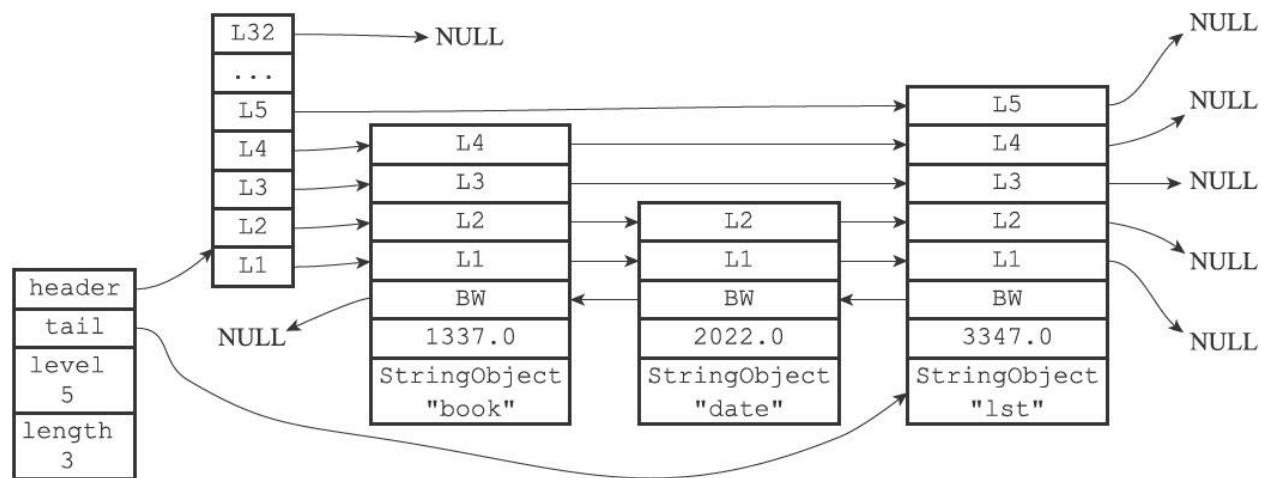
图17-23 节点7000的slots_to_keys跳跃表
