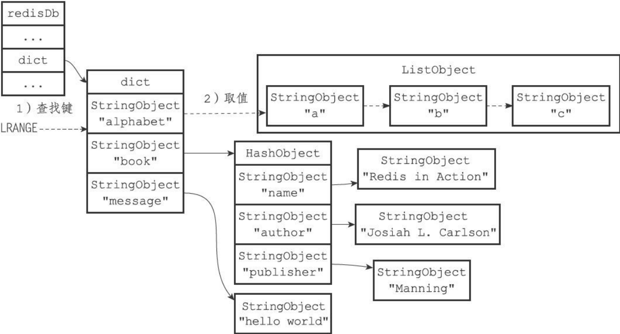
图9-10 使用LRANGE命令取值的过程
