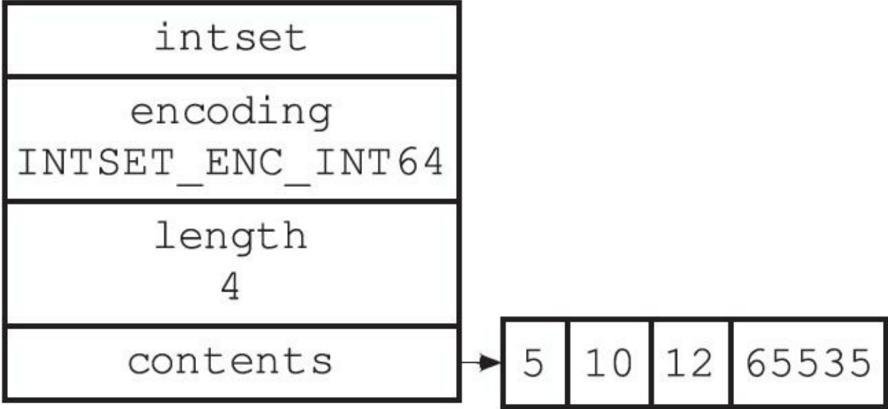
图6-12 删除4 294 967 295的整数集合
