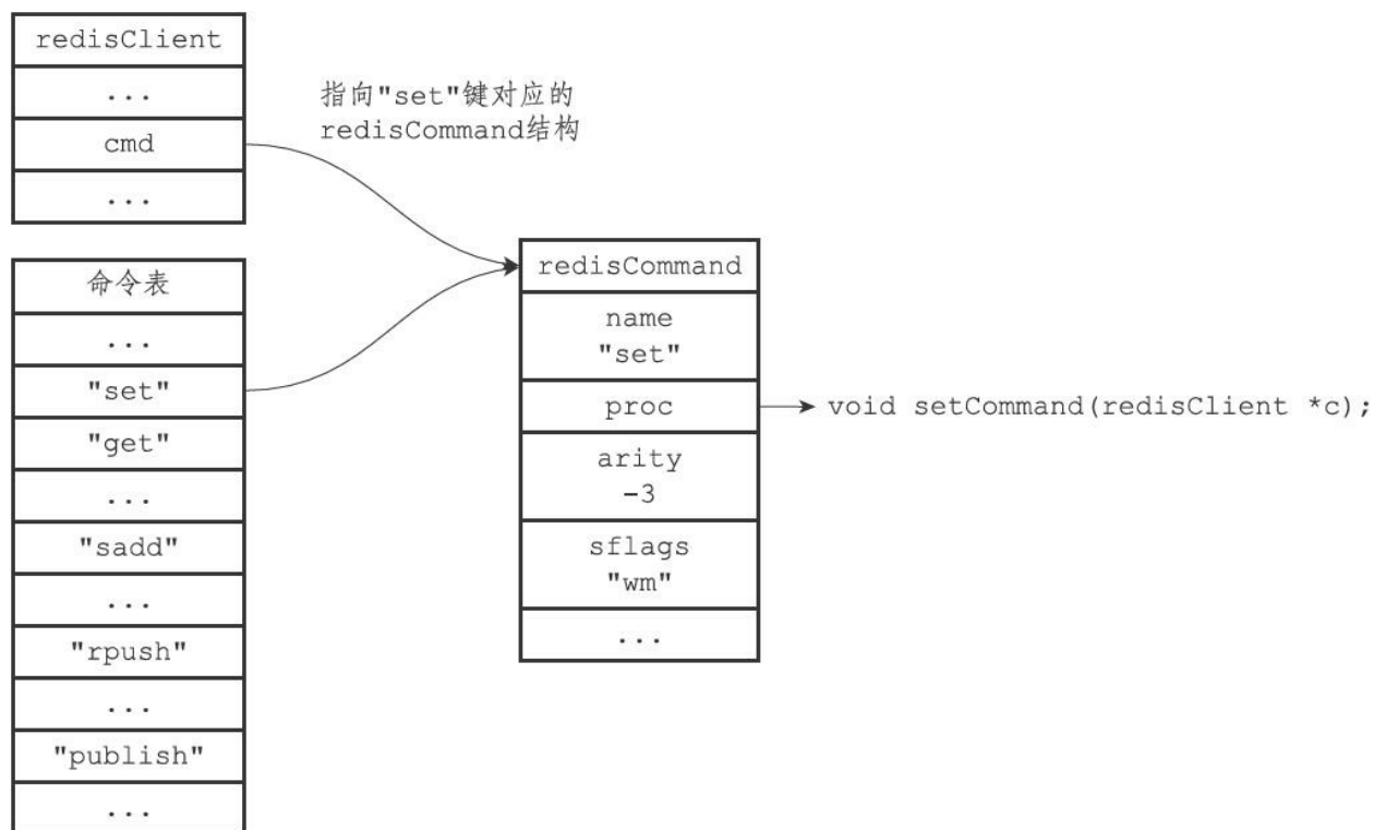
图14-5 设置客户端状态的cmd指针
