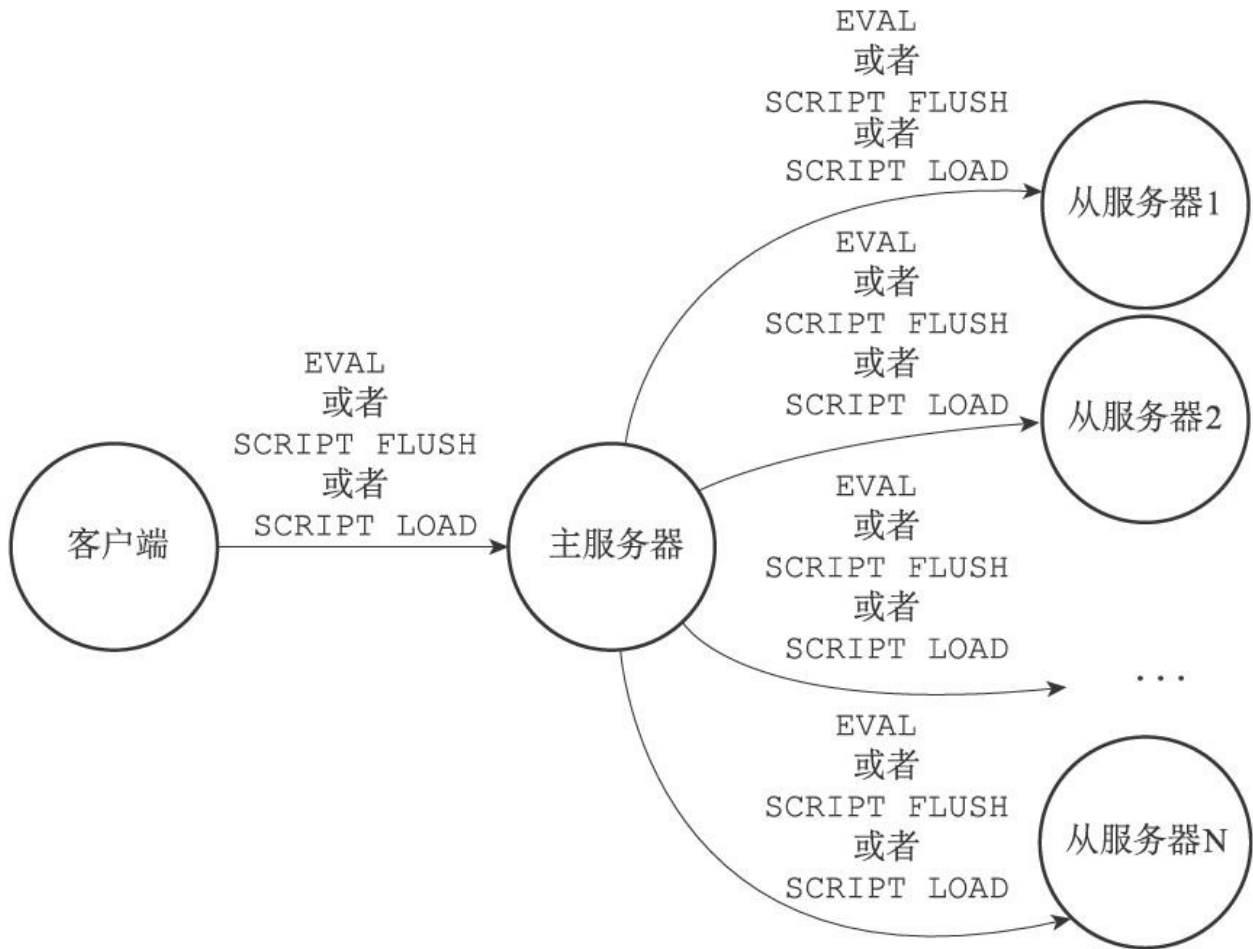
图20-9 将脚本命令传播给从服务器
