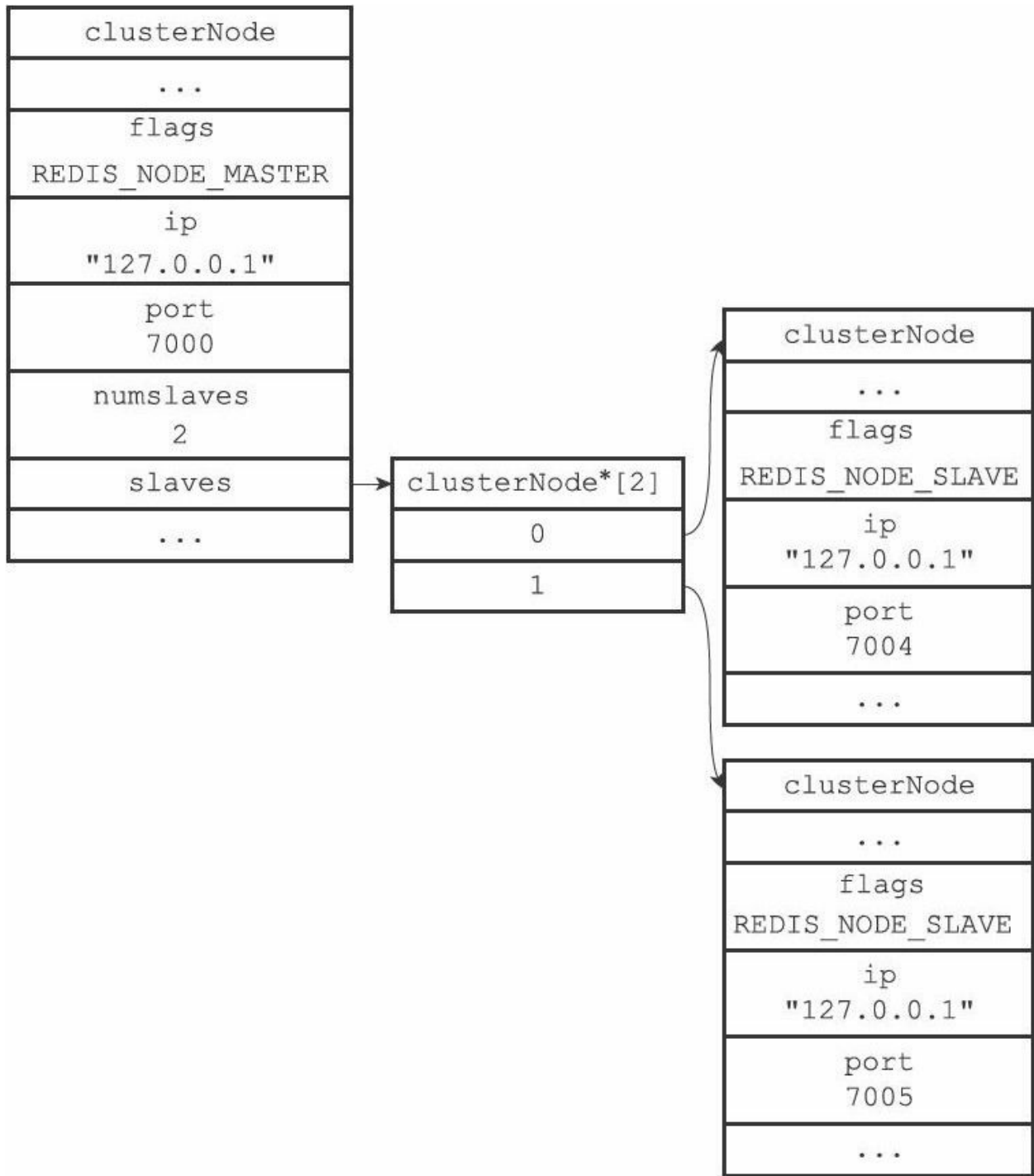
图17-36 集群中的各个节点为节点7000创建的clusterNode结构
