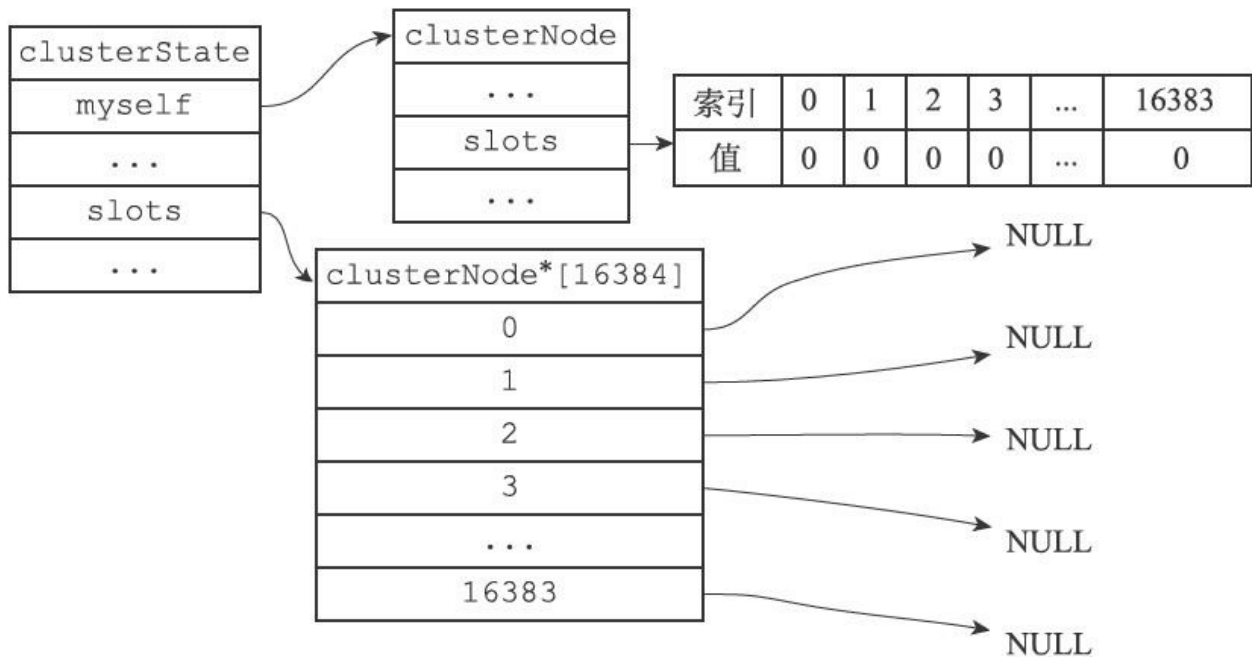
图17-16 节点的clusterState结构
