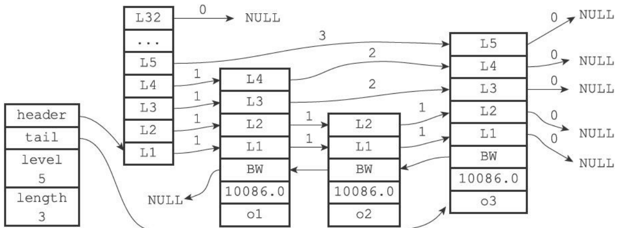
图5-7 三个带有相同分值的跳跃表节点
