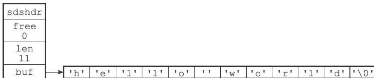
图2-6 11字节长的SDS
