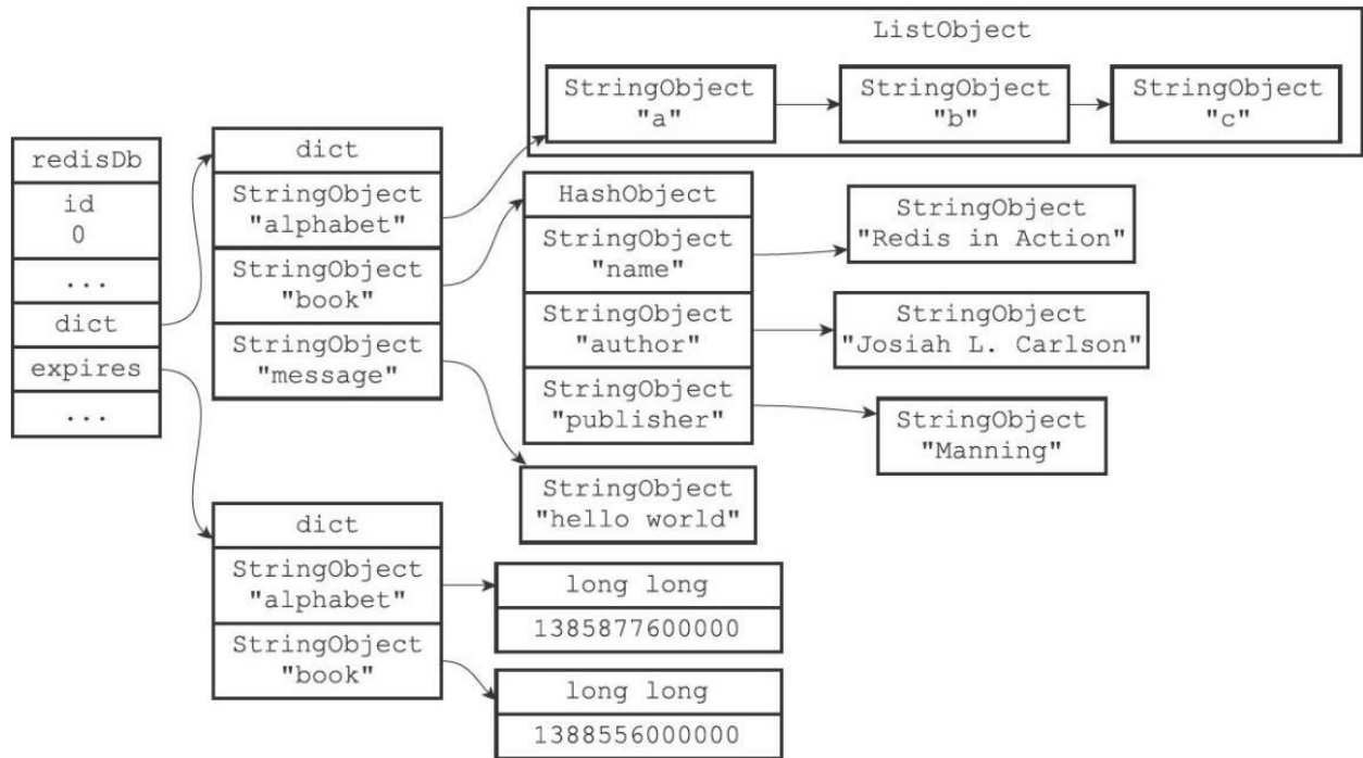
图11-3 一个数据库
