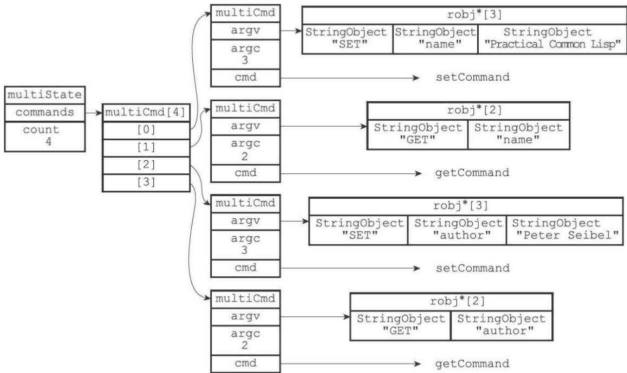
图19-2 事务状态
