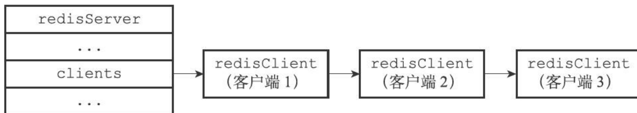
图13-2 clients链表
