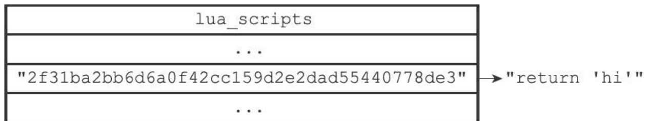
图20-7 lua_scripts字典
