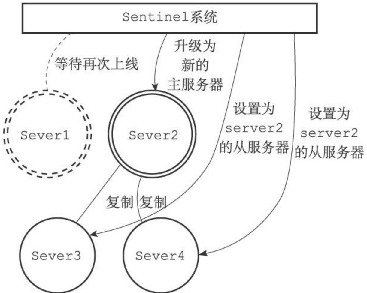
图16-3 故障转移
