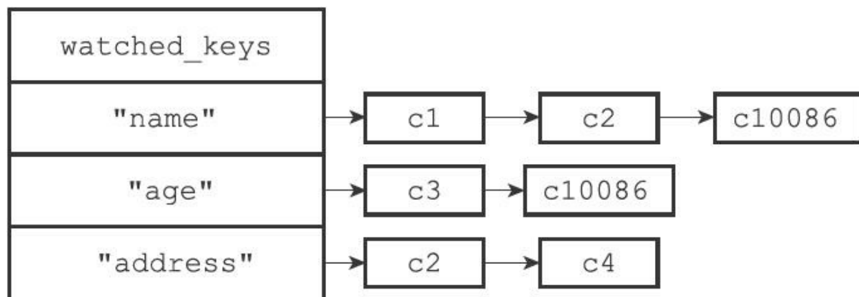
图19-5 watched_keys字典
