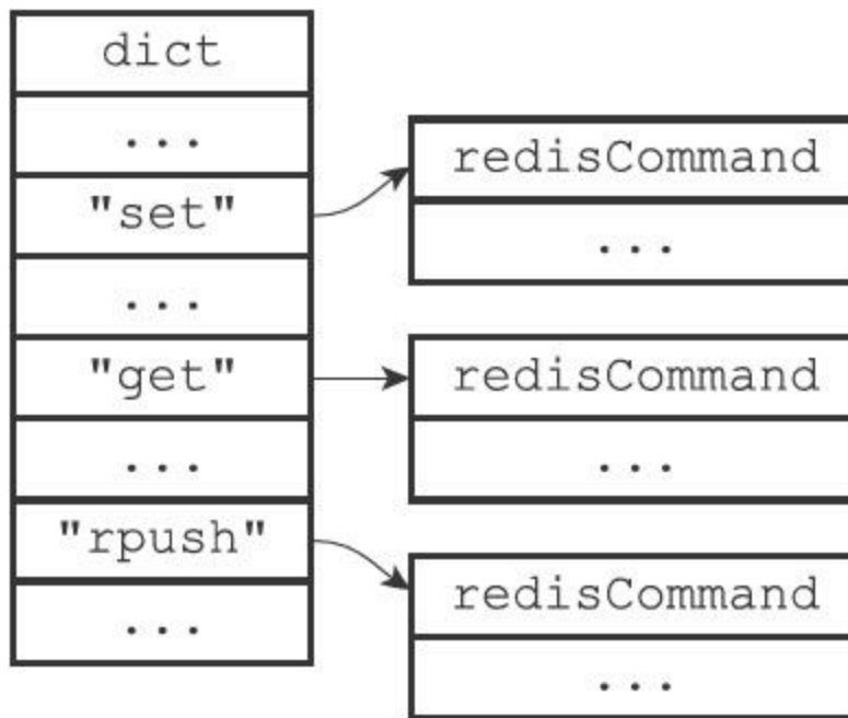
图13-6 命令表
