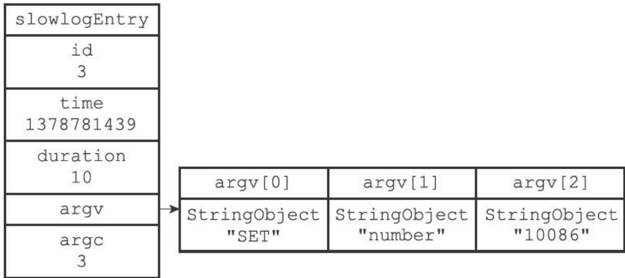
图23-1 slowlogEntry结构示例
