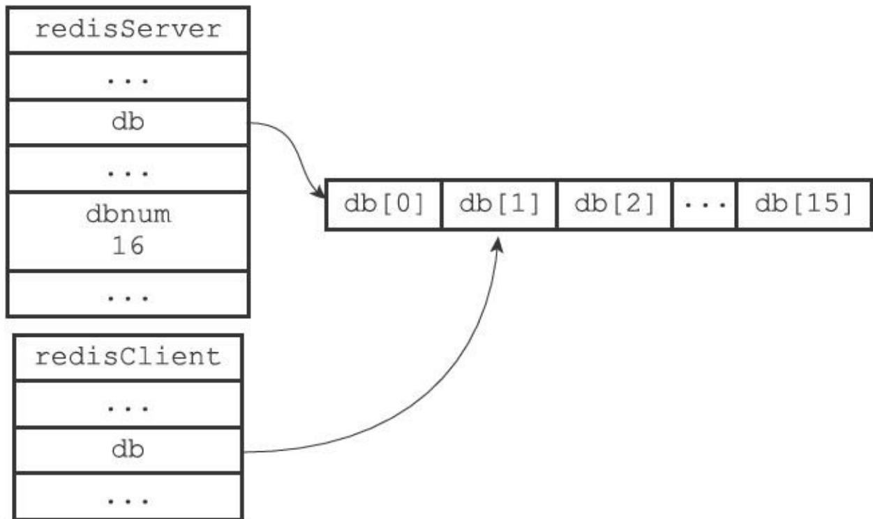
图9-2 客户端的目标数据库为1号数据库
