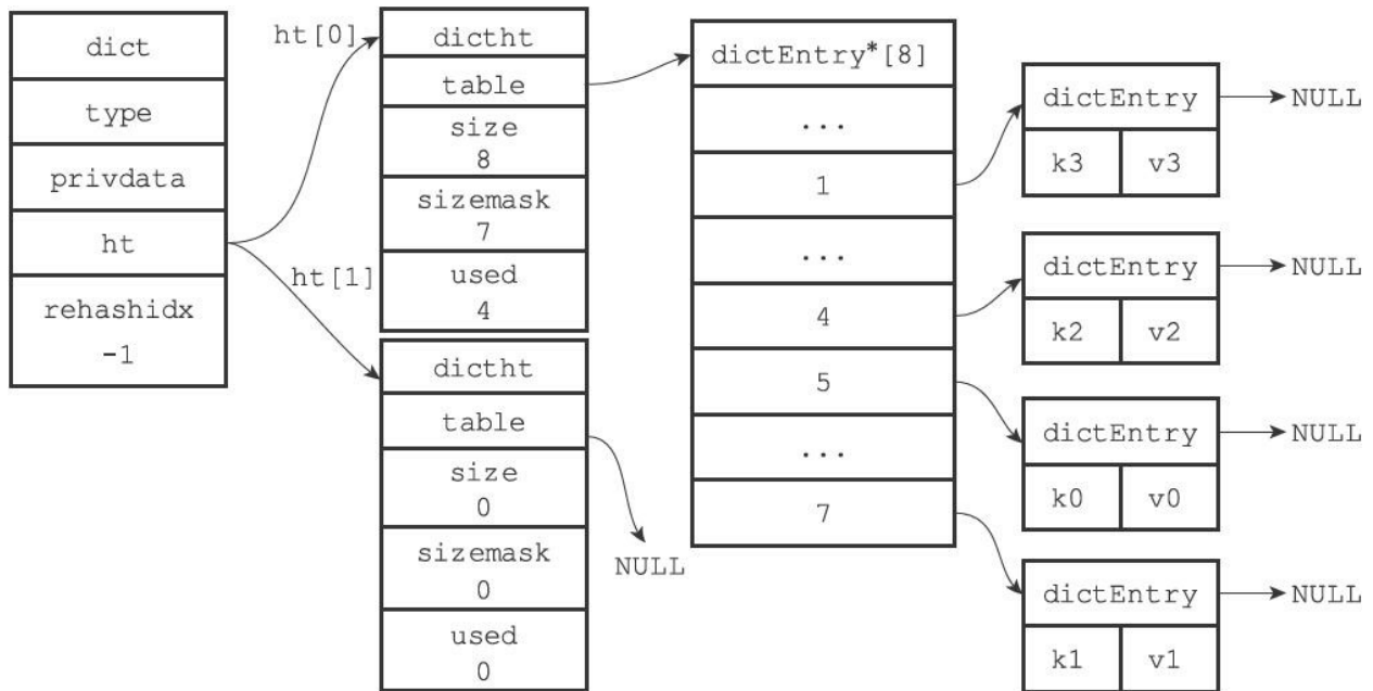
图4-17 rehash执行完毕
