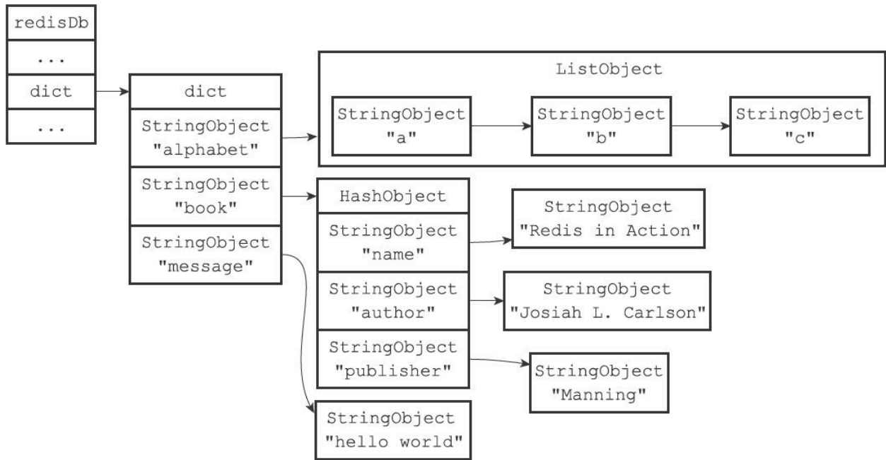
图9-4 数据库键空间例子
