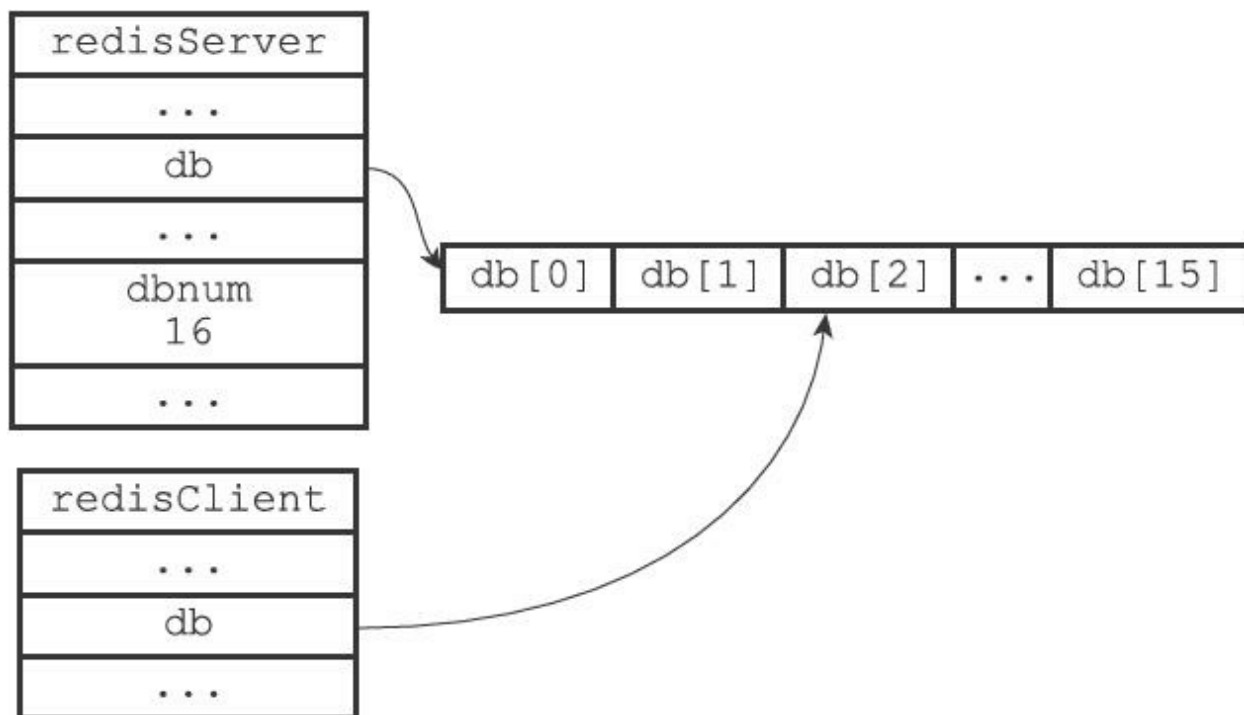
图9-3 客户端的目标数据库为2号数据库
