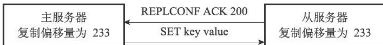
图15-25 主服务器向从服务器补发缺失的数据
