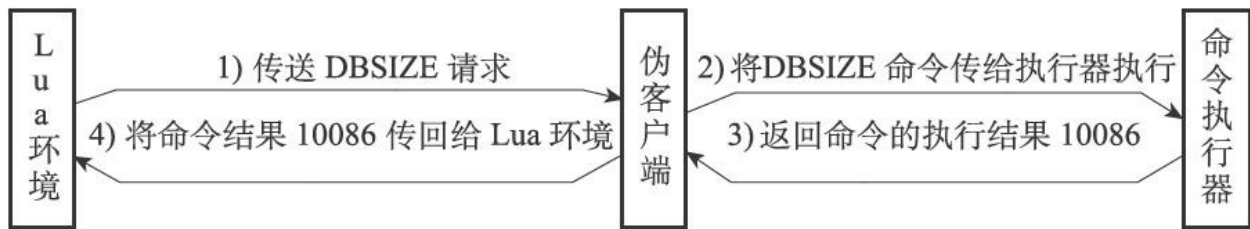
图20-3 Lua脚本执行DBSIZE命令时的通信步骤
