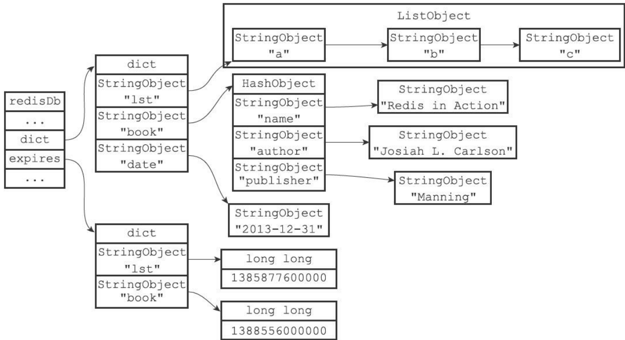
图17-22 节点7000的数据库
