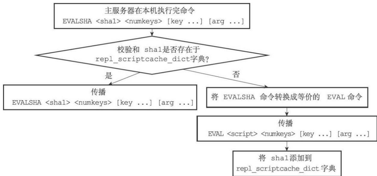
图20-12 主服务器判断传播EVAL还是EVALSHA的过程
