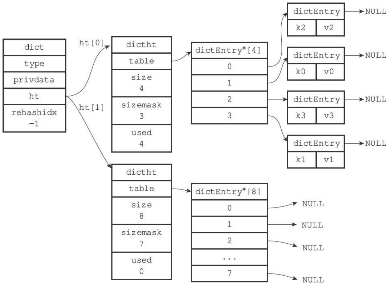
图4-12 准备开始rehash
