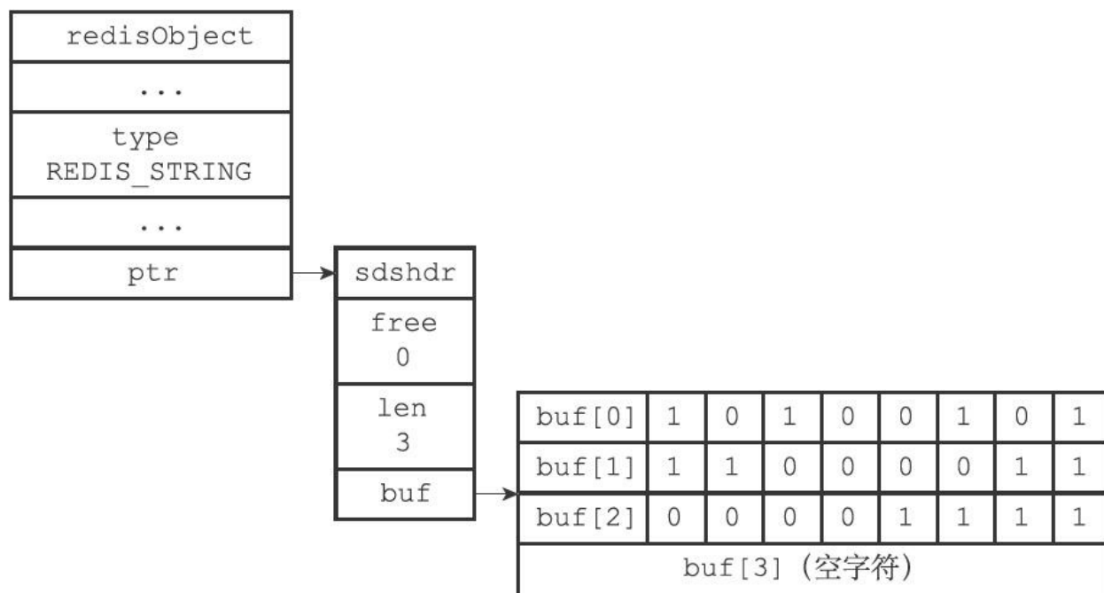
图22-3 三字节长的位数组的SDS表示
