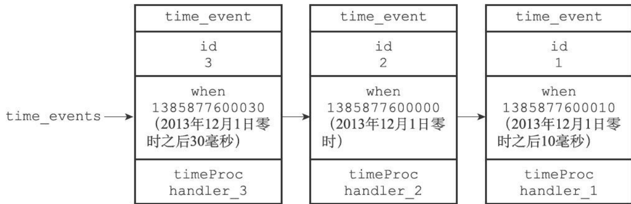
图12-8 用链表连接起来的三个时间事件
