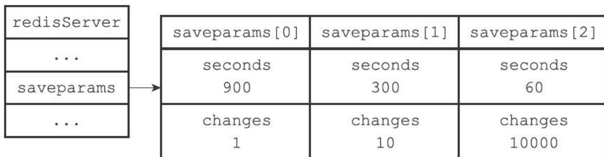
图10-6 服务器状态中的保存条件
