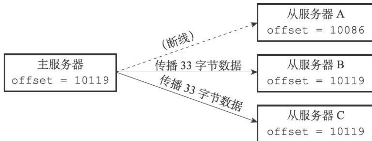
图15-9 因为断线而处于不一致状态的从服务器A
