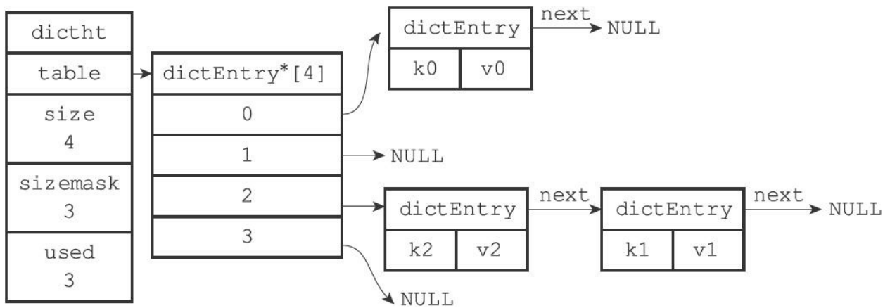
图4-7 使用链表解决k2和k1的冲突
