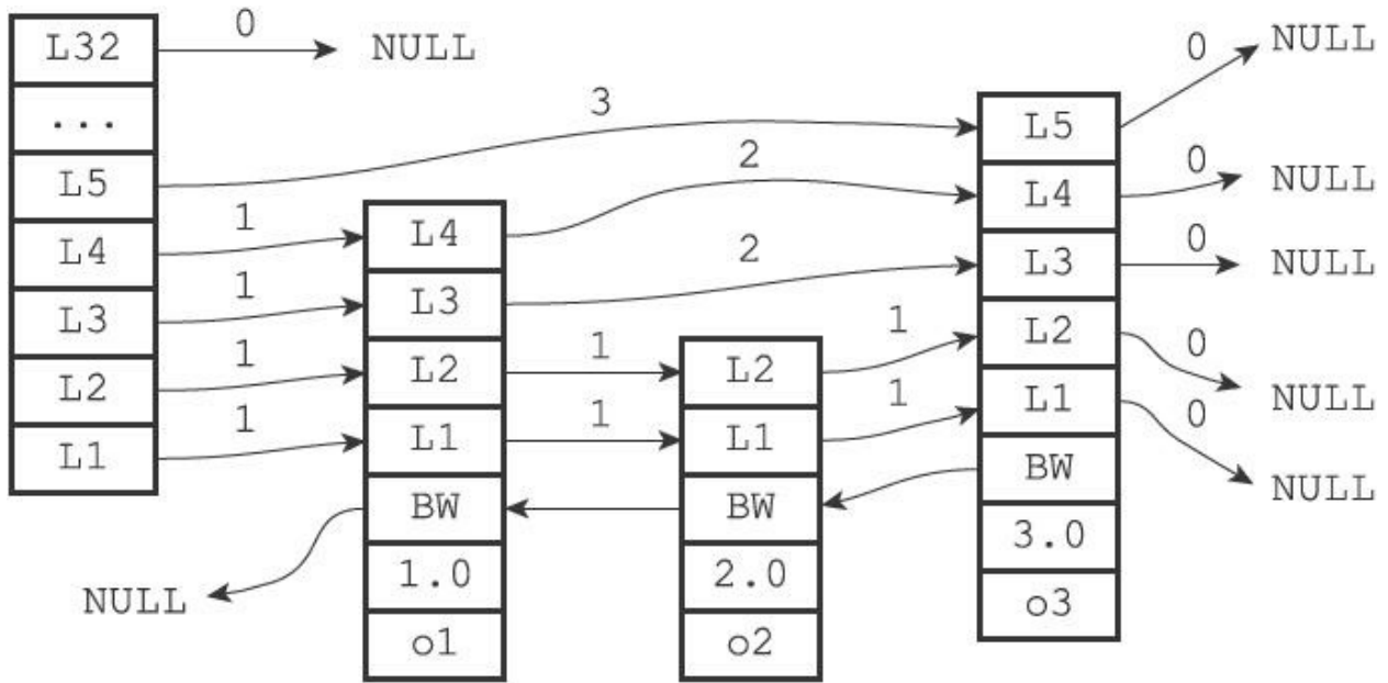
图5-8 由多个跳跃节点组成的跳跃表
