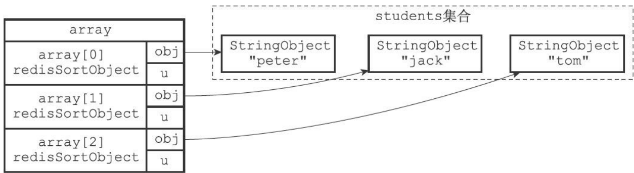
图21-17 排序之前的数组
