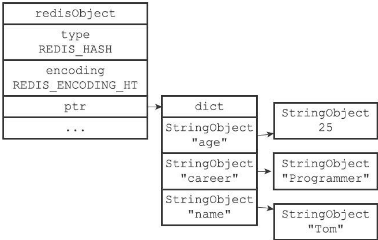
图8-11 hashtable编码的profile哈希对象
