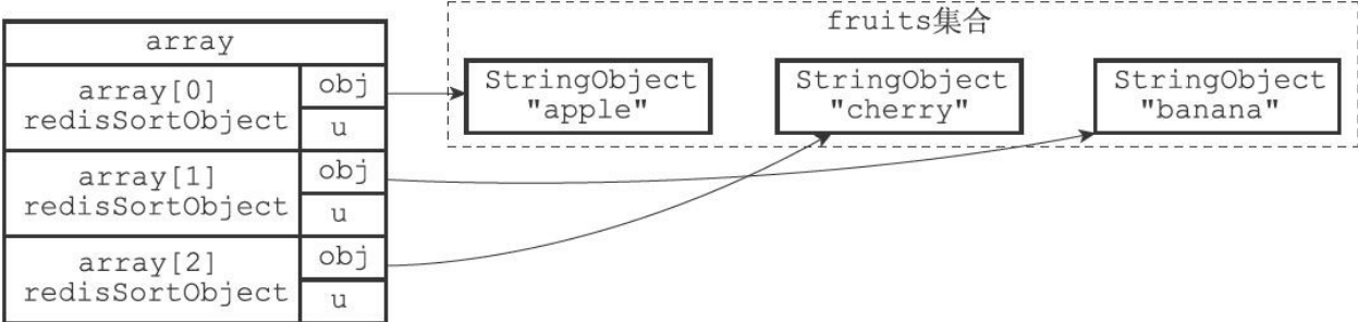
图21-6 按集合元素进行排序后的数组
