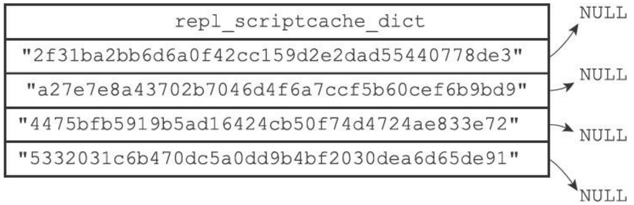
图20-14 执行EVALSHA命令之后的repl_scriptcache_dict字典
