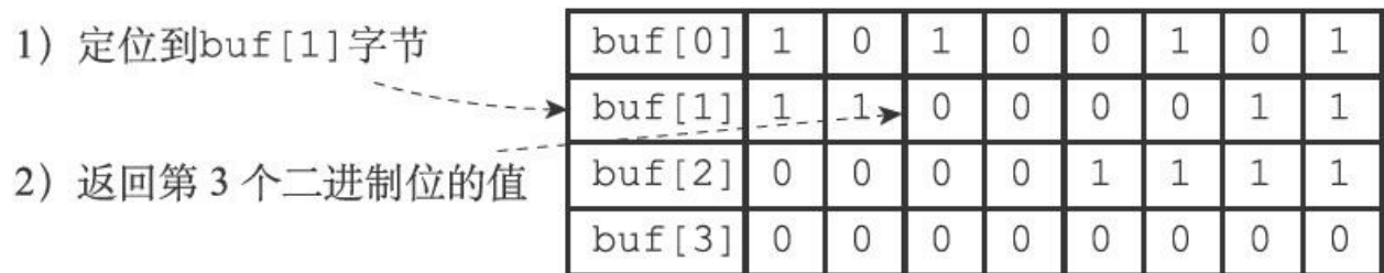
图22-5 查找并返回offset为10的二进制位的过程
