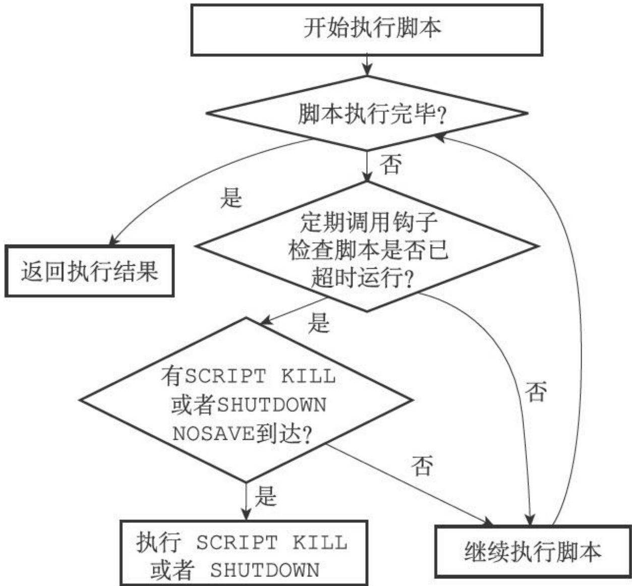
图20-8 带有超时处理钩子的脚本的执行过程
