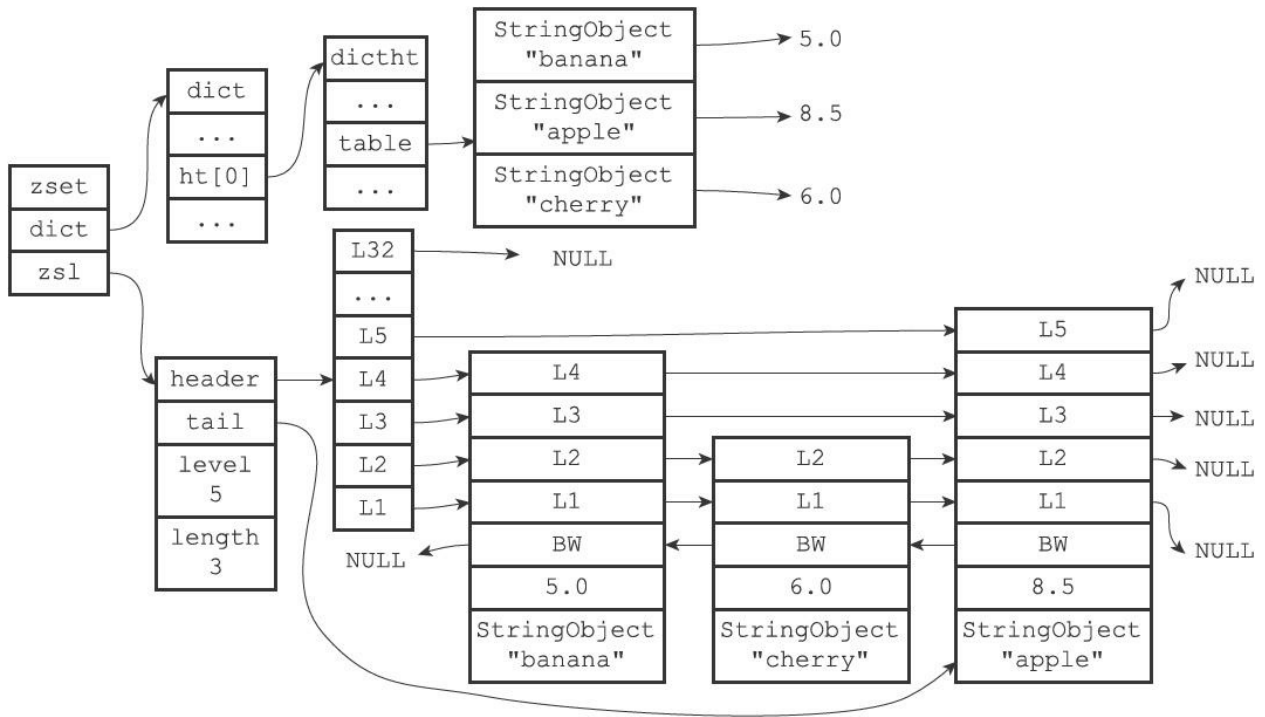
图8-17 有序集合元素同时被保存在字典和跳跃表中
