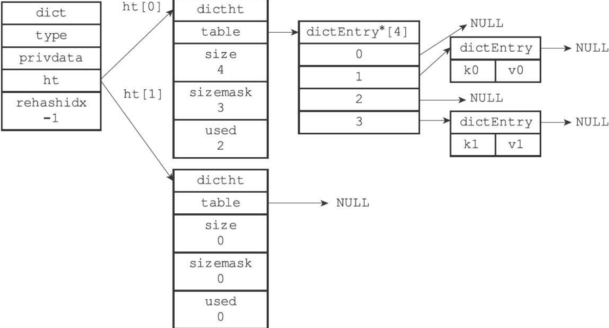
图4-3 普通状态下的字典
