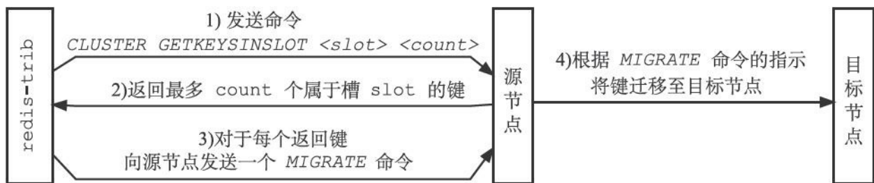
图17-24 迁移键的过程
