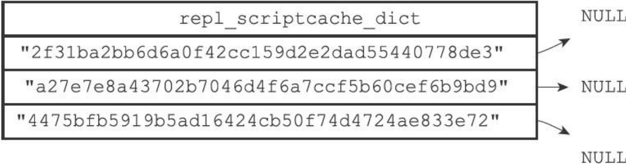
图20-10 一个repl_scriptcache_dict字典示例
