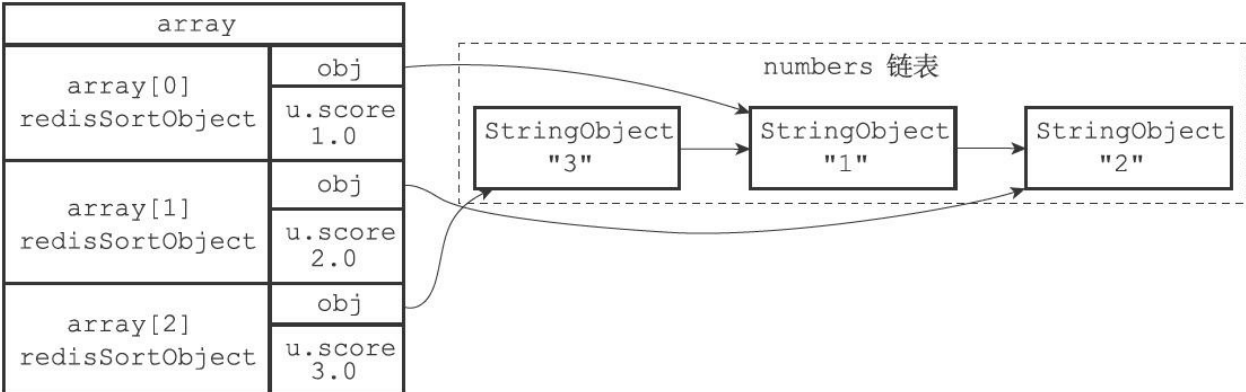
图21-3 设置数组项的u.score属性
