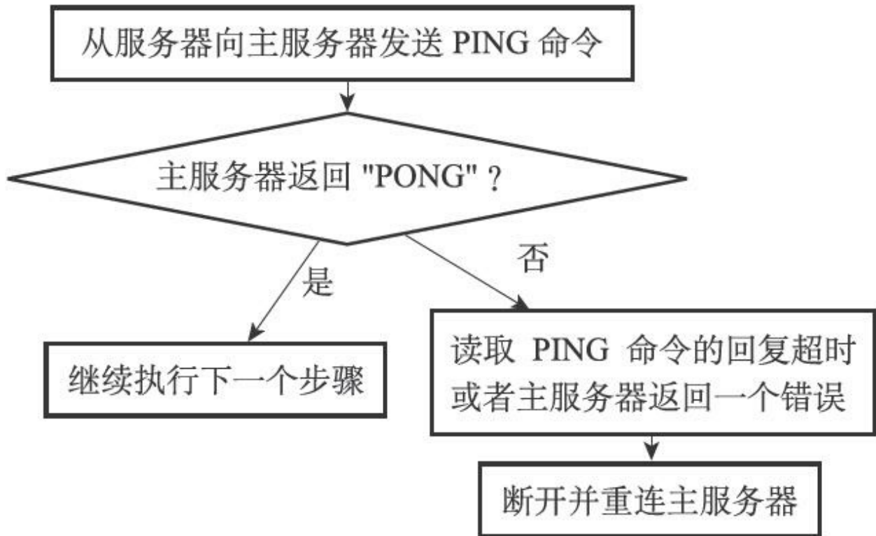
图15-17 从服务器在发送PING命令时可能遇到的情况
