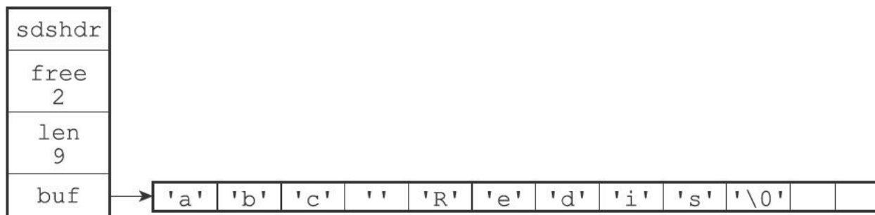
图2-16 执行sdscat之后的SDS
