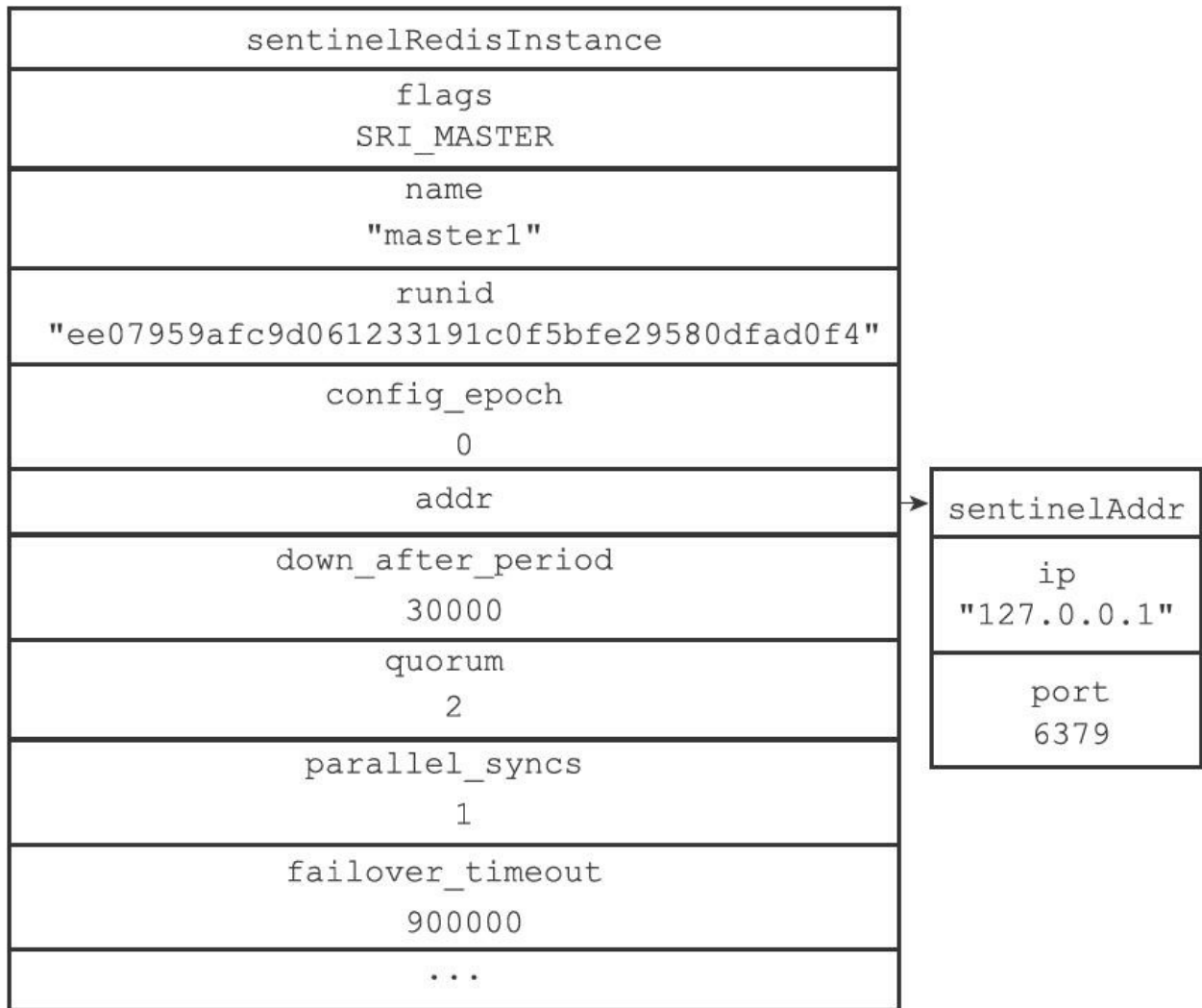
图16-5 master1的实例结构
