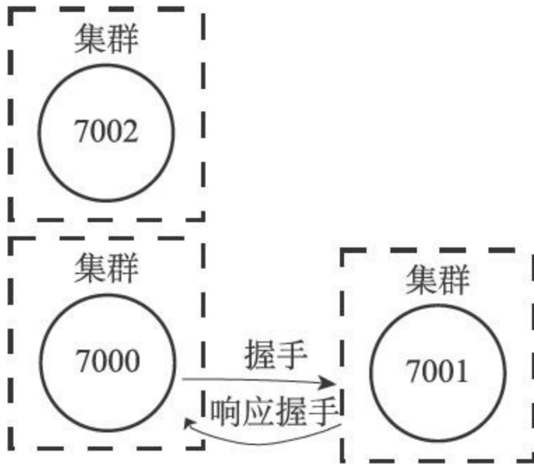
图17-2 节点7000和7001进行握手
