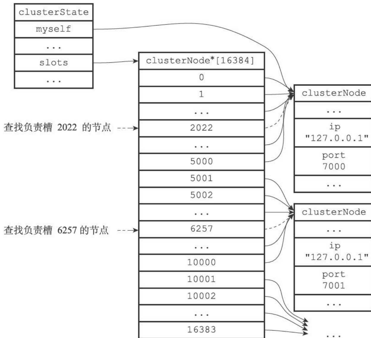
图17-19 节点7000的clusterState结构
