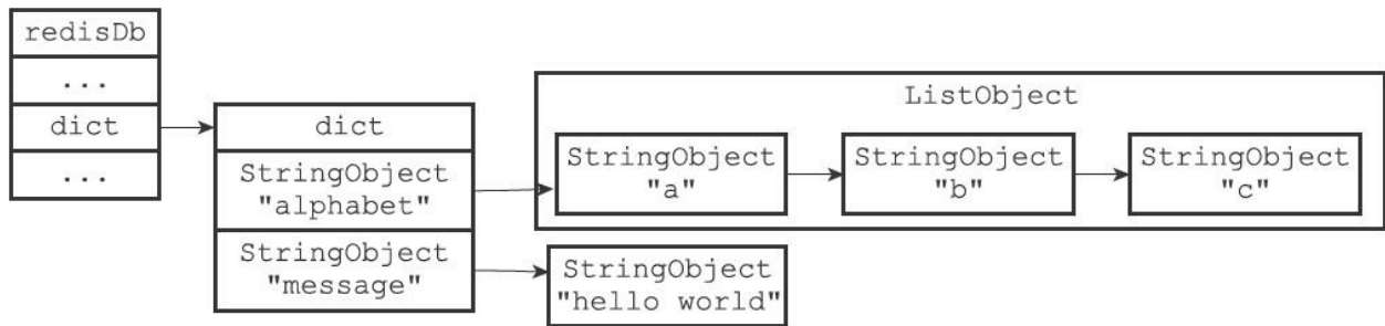
图9-6 删除book键之后的键空间
