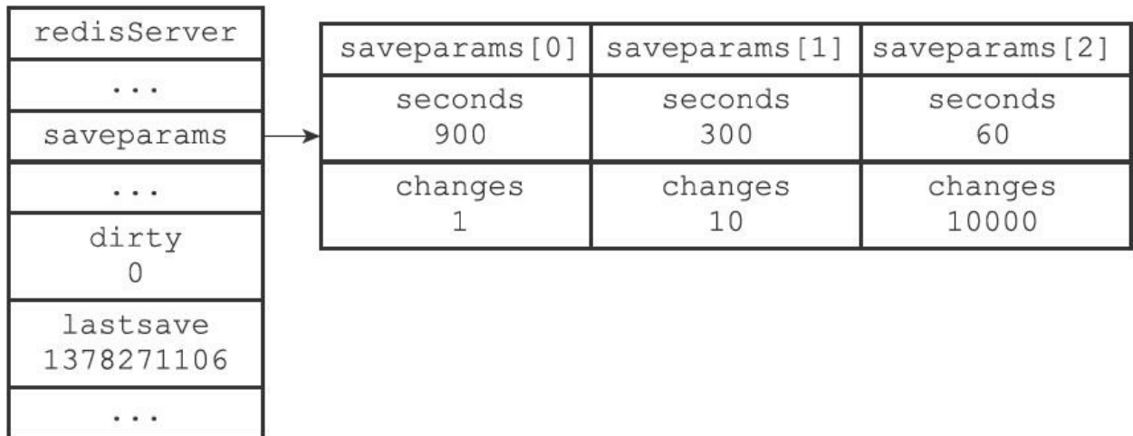
图10-9 执行BGSAVE之后的服务器状态
