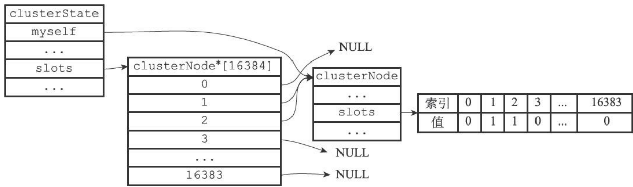
图17-17 执行CLUSTER ADDSLOTS命令之后的clusterState结构
