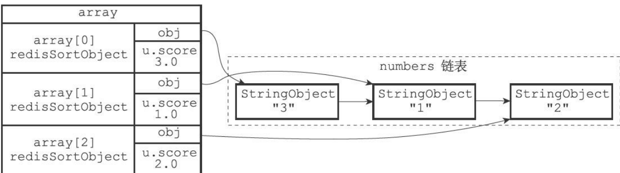
图21-3 设置数组项的u.score属性
