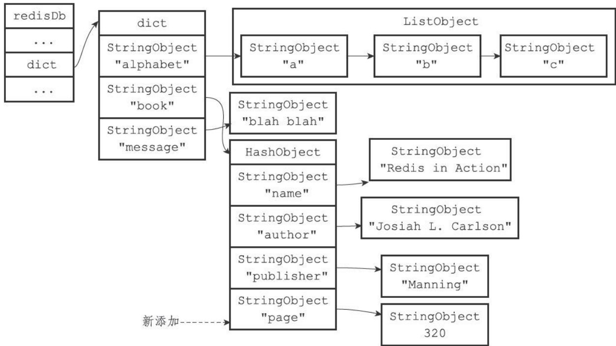
图9-8 使用HSET更新book键
