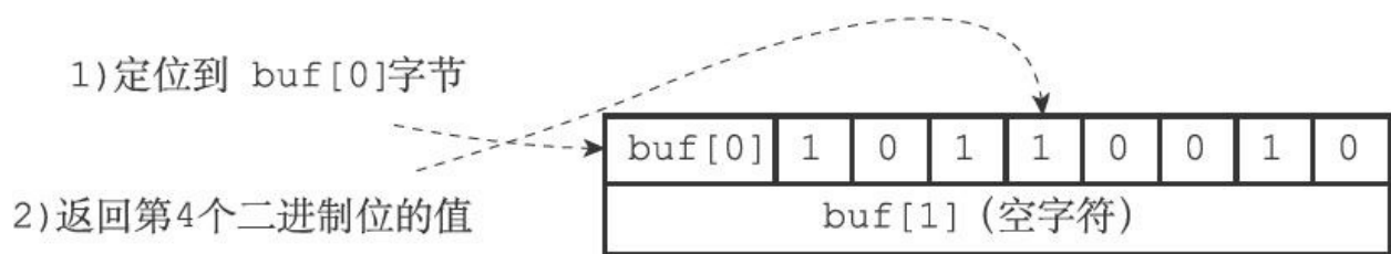
图22-4 查找并返回offset为3的二进制位的过程
