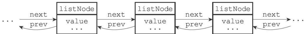
图3-1 由多个listNode组成的双端链表
