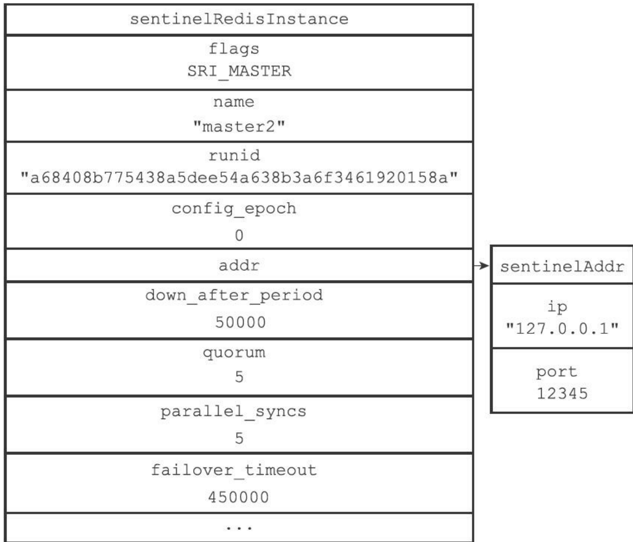
图16-6 master2的实例结构
