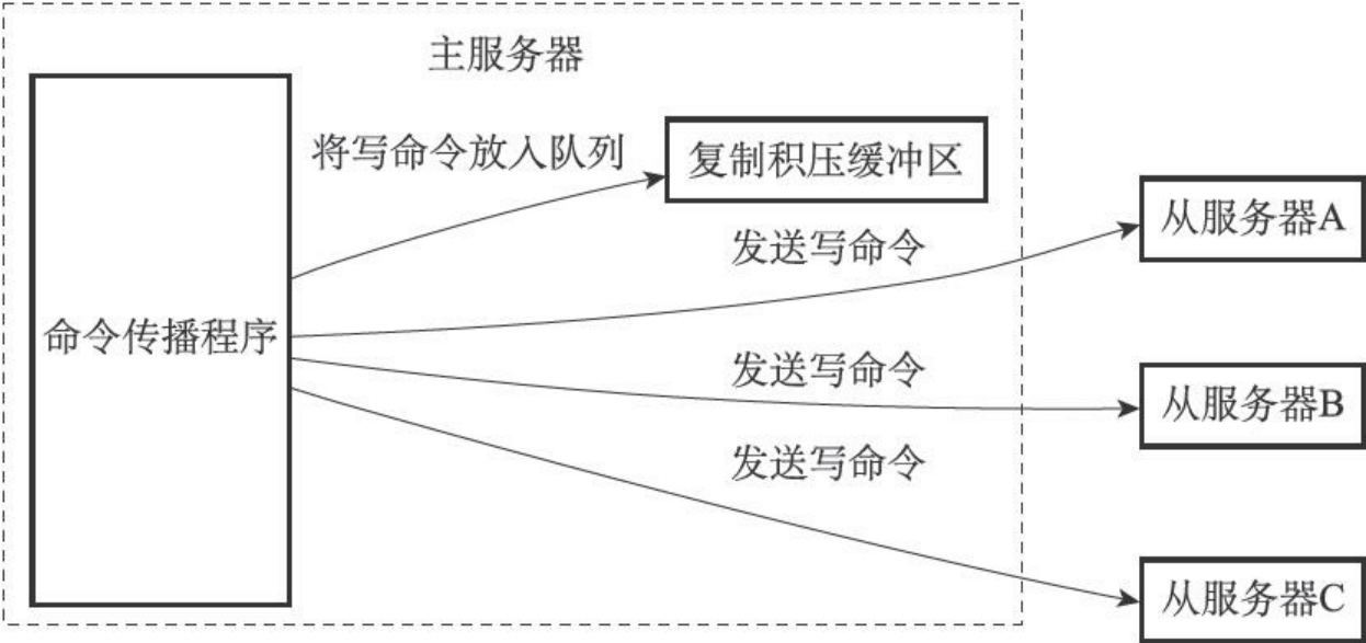
图15-10 主服务器向复制积压缓冲区和所有从服务器传播写命令数据
