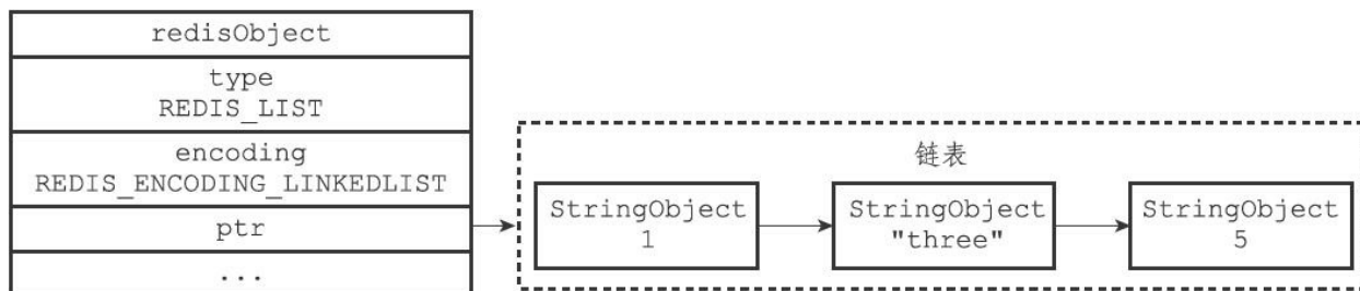
图8-6 linkedlist编码的numbers列表对象
