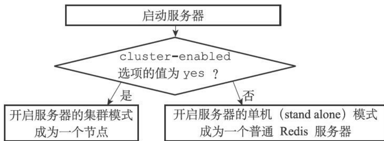
图17-6 服务器判断是否开启集群模式的过程
