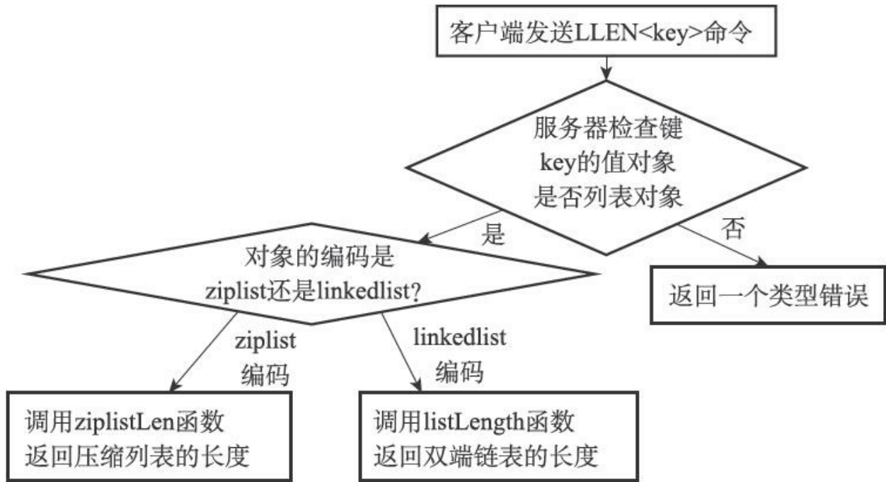
图8-19 LLEN命令的执行过程
