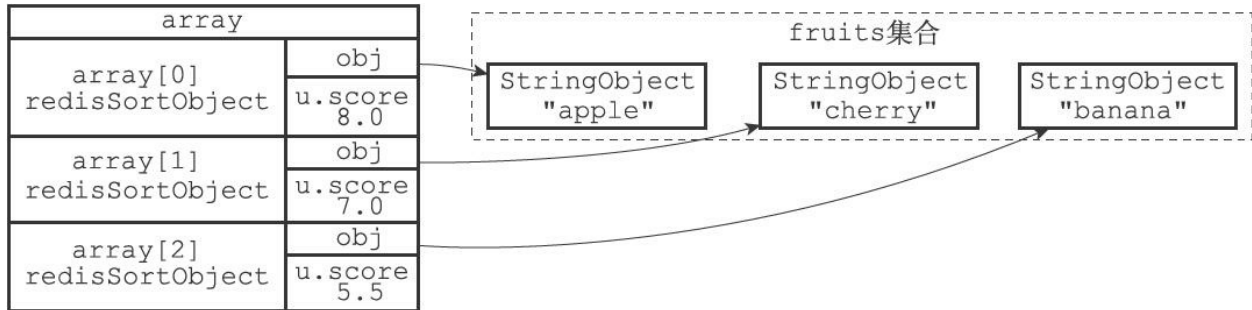
图21-10 根据权重键的值设置数组项的u.score属性
