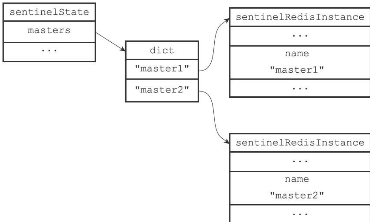
图16-7 Sentinel状态以及masters字典
