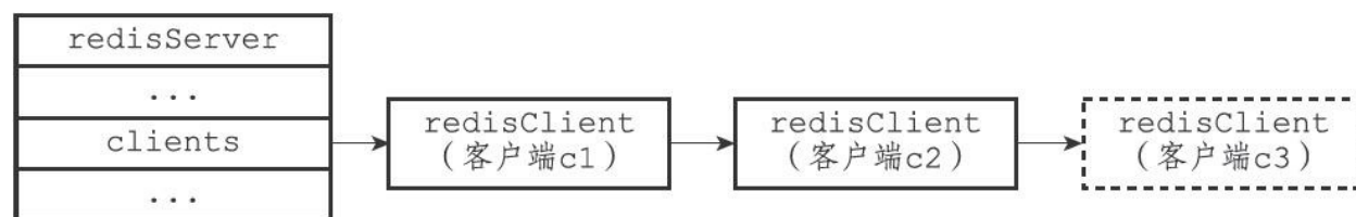
图13-12 服务器状态结构的clients链表
