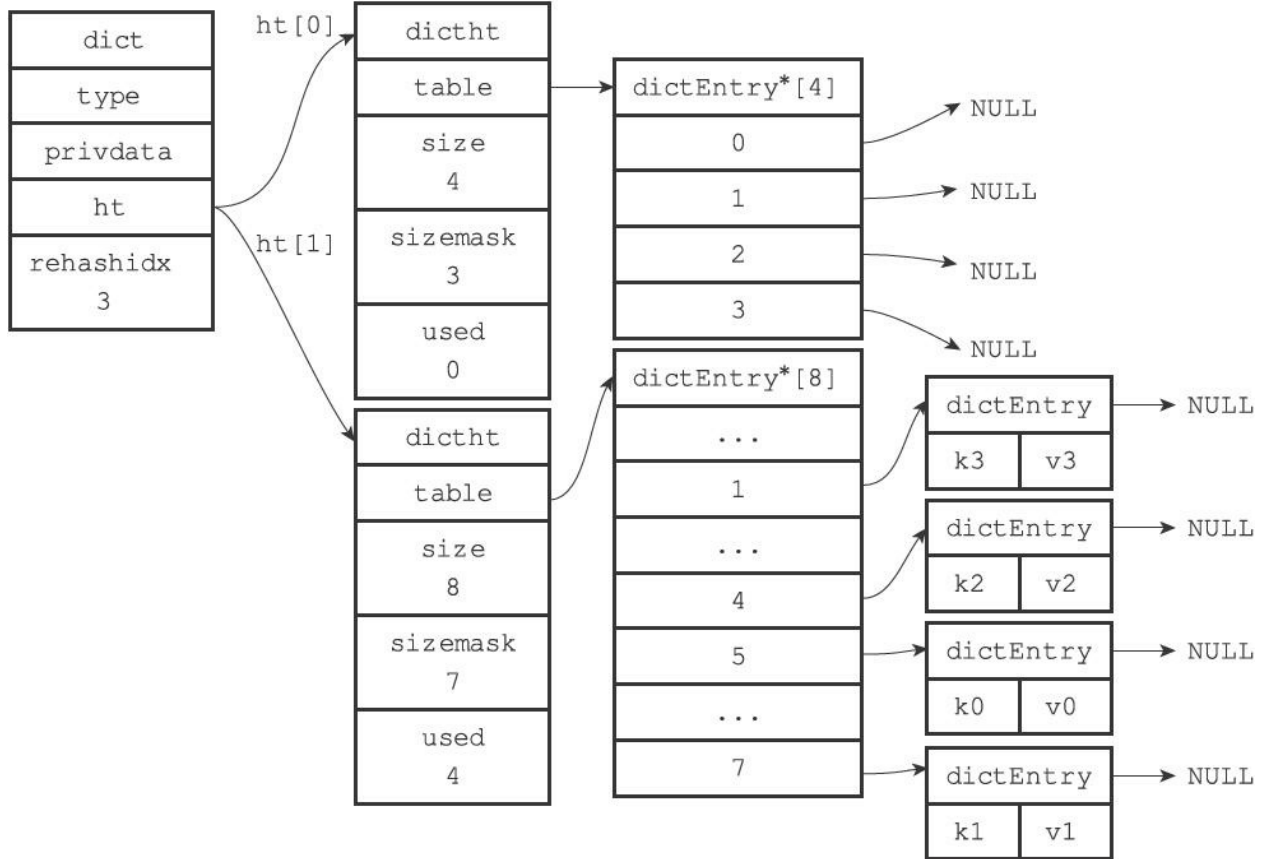
图4-16 rehash索引3上的键值对
