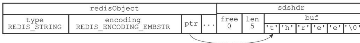
图8-8 完整的字符串对象表示
