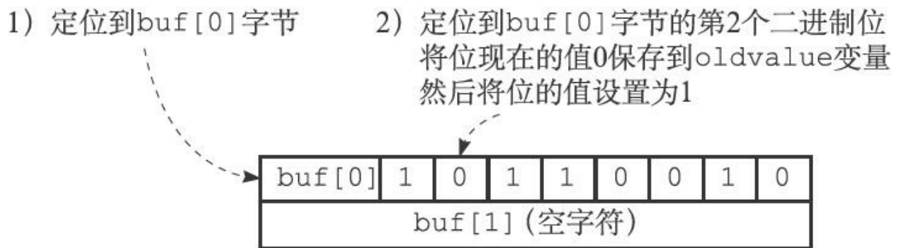
图22-6 SETBIT命令的执行过程
