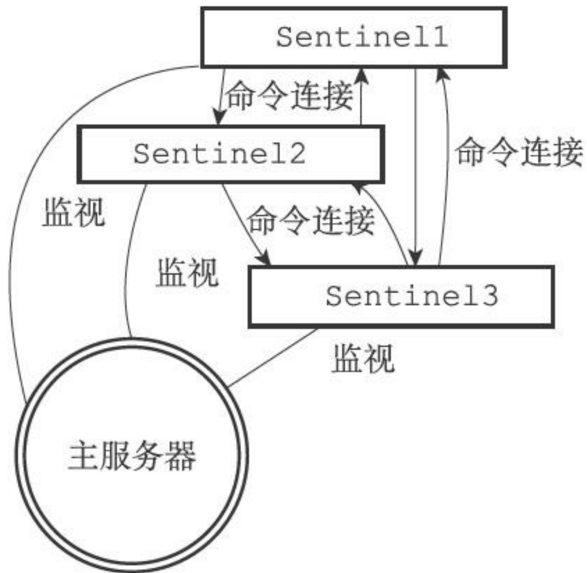
图16-16 各个Sentinel之间的网络连接
