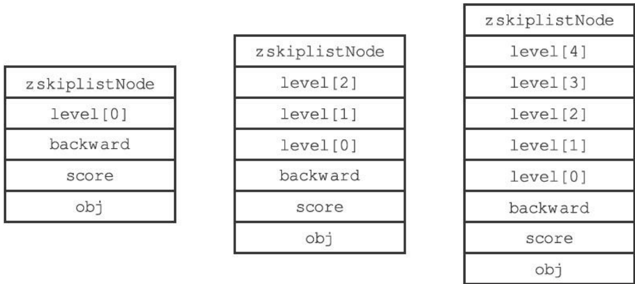
图5-2 带有不同层高的节点
