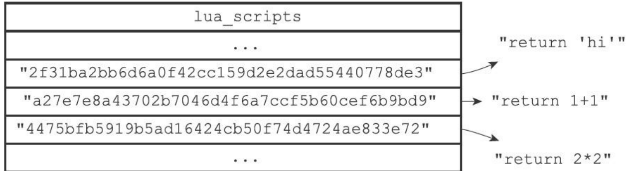
图20-4 lua_scripts字典示例
