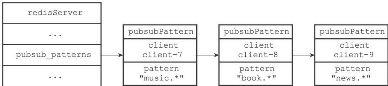
图18-14 执行PUNSUBSCRIBE命令之前的pubsub_patterns链表
