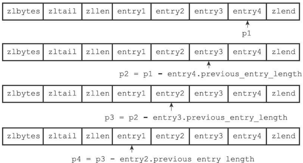
图7-8 一个从表尾向表头遍历的例子
