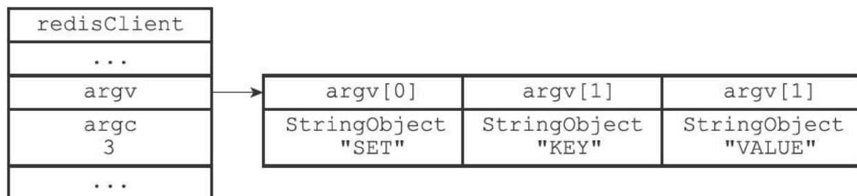
图14-3 客户端状态的argv属性和argc属性
