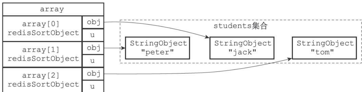
图21-17 排序之前的数组
