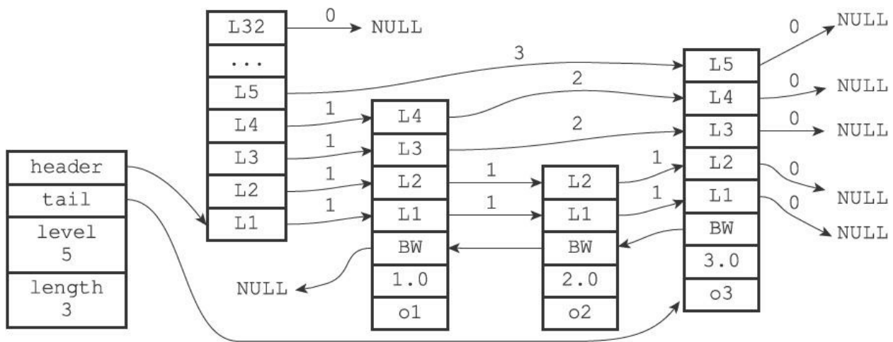
图5-1 一个跳跃表
