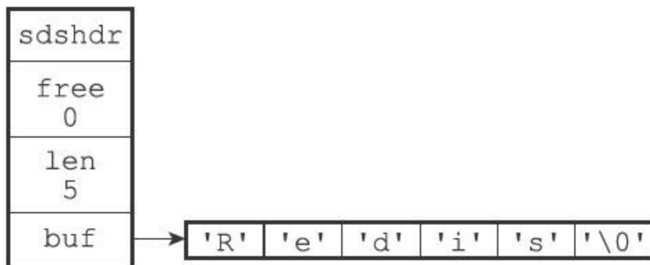
图2-1 SDS示例
