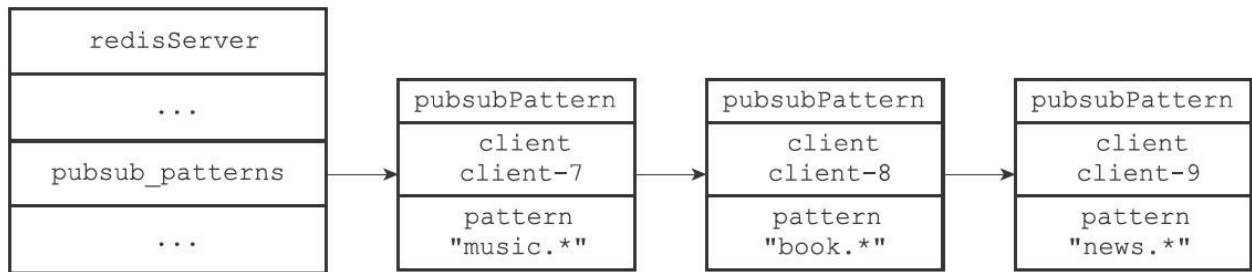
图18-20 pubsub_patterns链表
