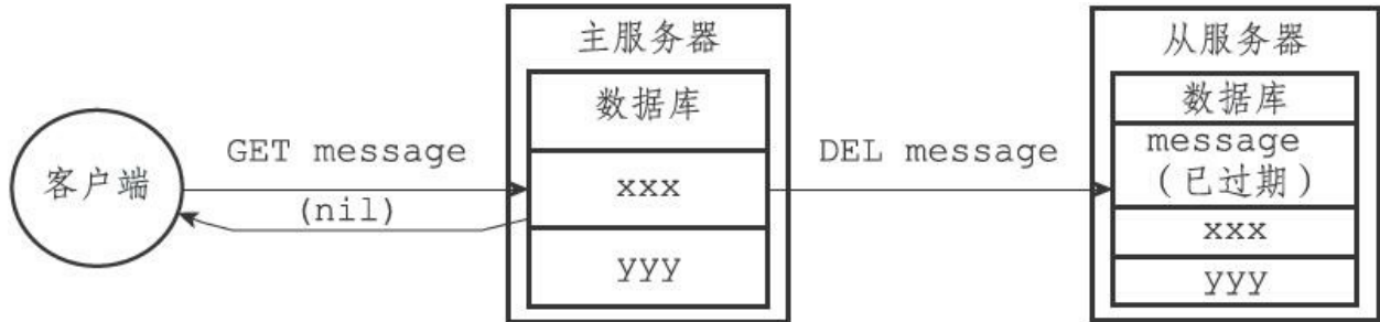
图9-19 主从服务器删除过期键 (3)
