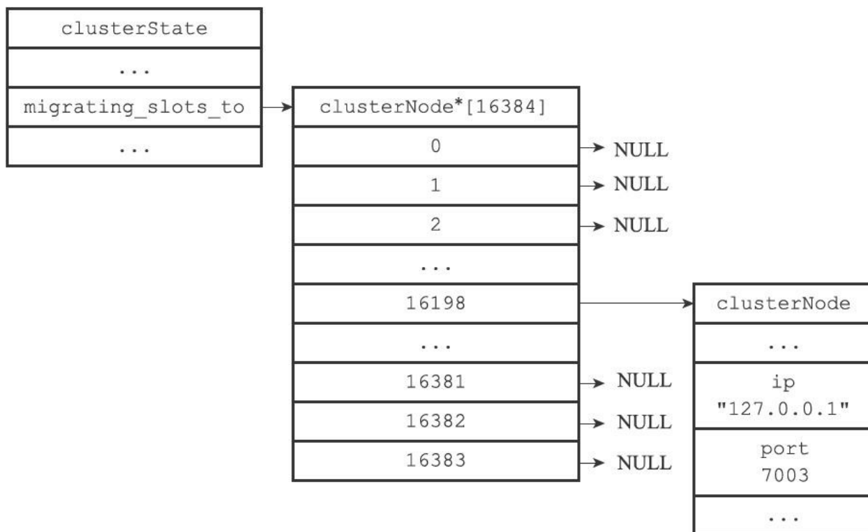
图17-28 节点7002的migrating_slots_to数组
