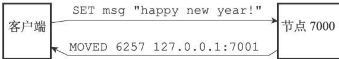
图17-20 节点7000向客户端返回MOVED错误
