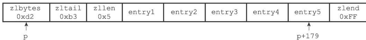
图7-3 包含五个节点的压缩列表
