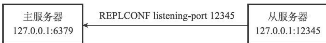
图15-20 从服务器向主服务器发送监听端口
