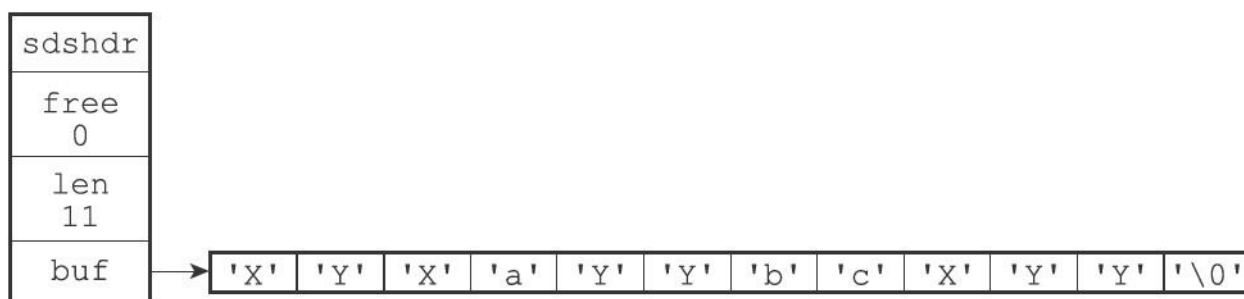
图2-14 执行sdstrim之前的SDS
