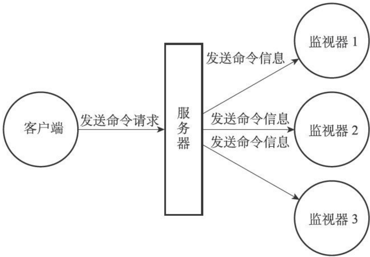
图24-1 命令的接收和信息的发送
