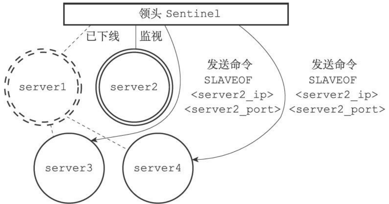
图16-24 让从服务器复制新的主服务器
