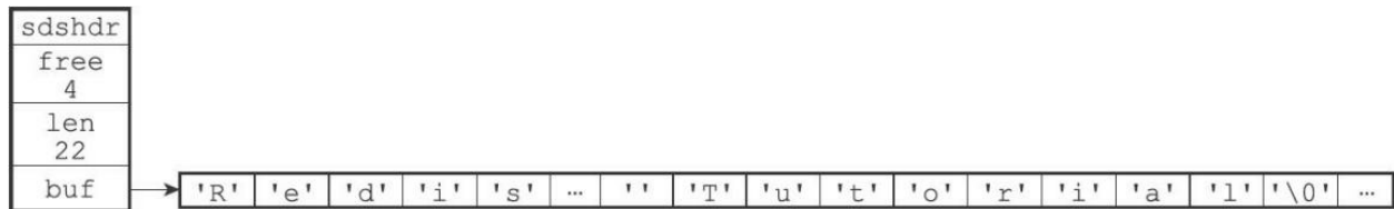
图2-13 再次执行sdscat之后的SDS
