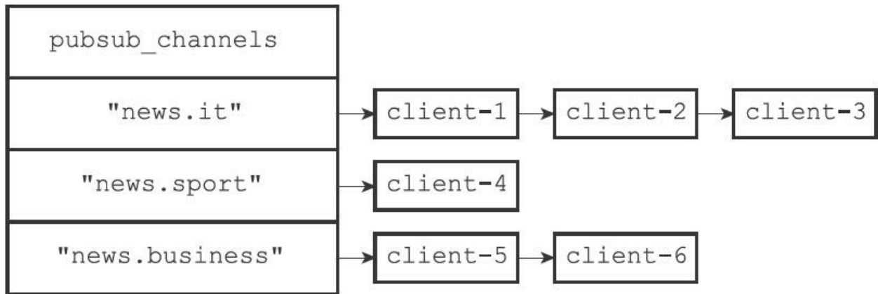
图18-6 一个pubsub_channels字典示例
