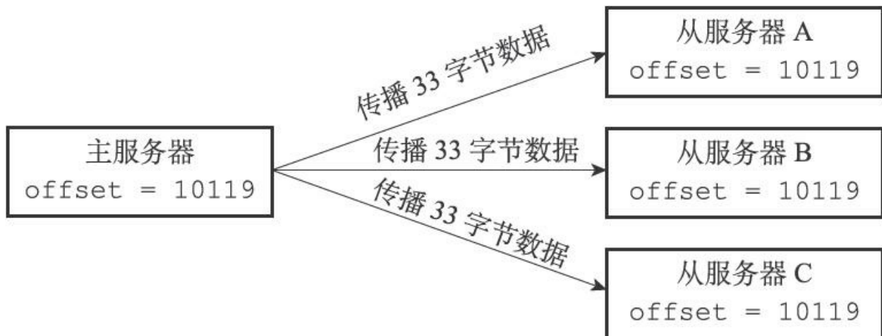
图15-8 更新偏移量之后的主从服务器
