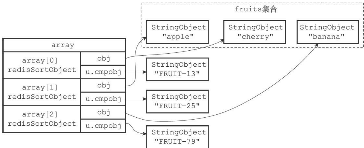
图21-14 按u.cmpobj所指向的字符串对象进行排序之后的数组
