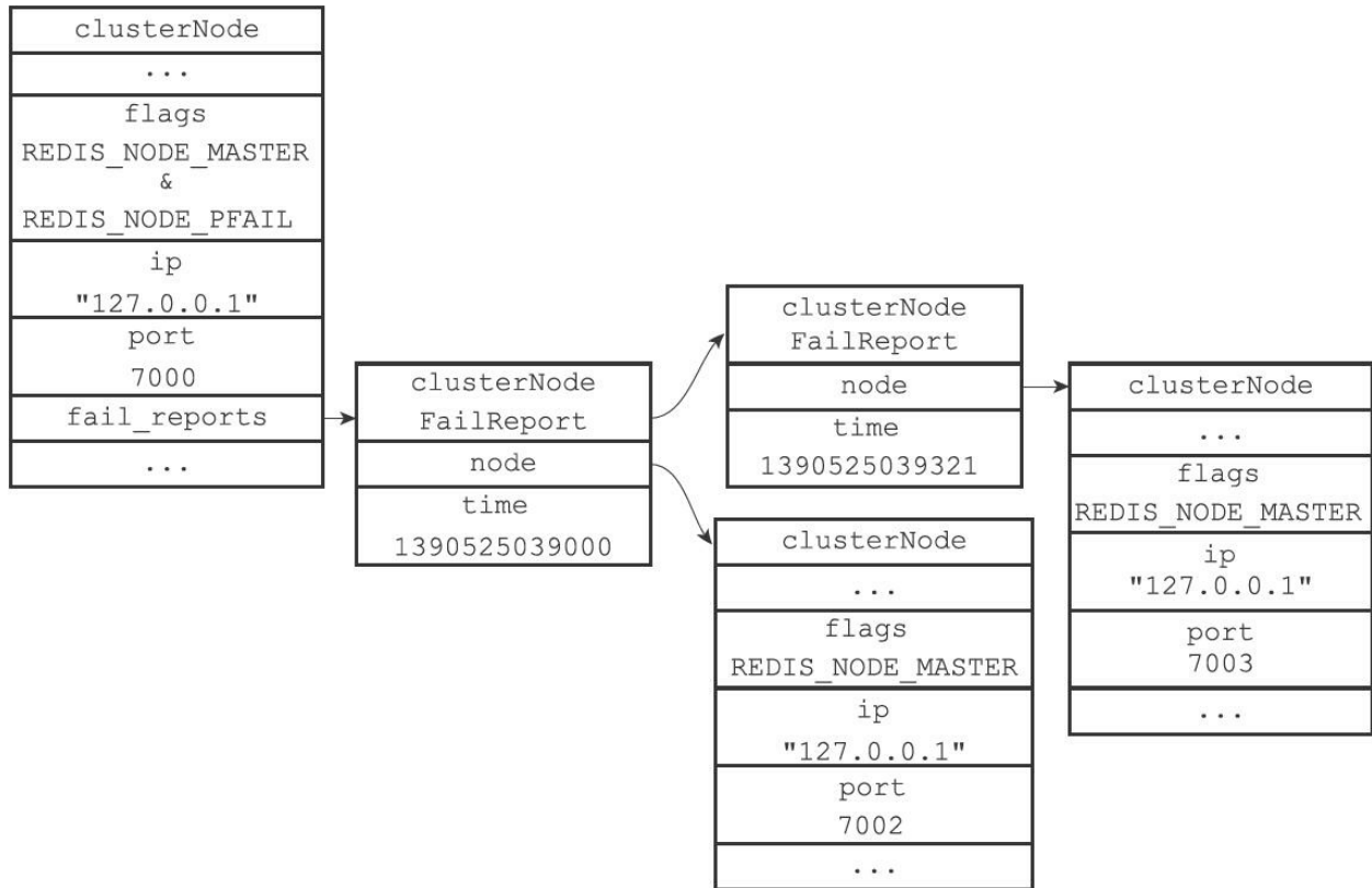
图17-38 节点7000的下线报告
