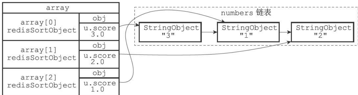
图21-8 执行降序排序的数组
