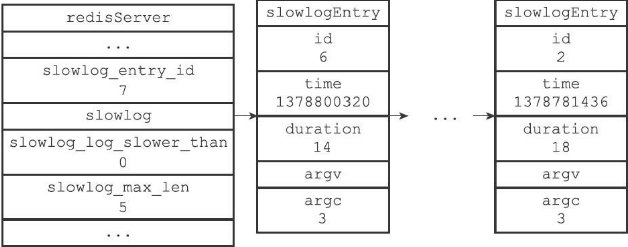
图23-4 删除id为1的慢查询日志之后的服务器状态
