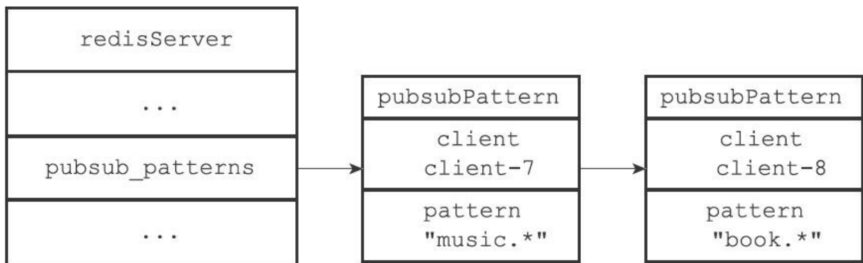
图18-15 执行PUNSUBSCRIBE命令之后的pubsub_patterns链表
