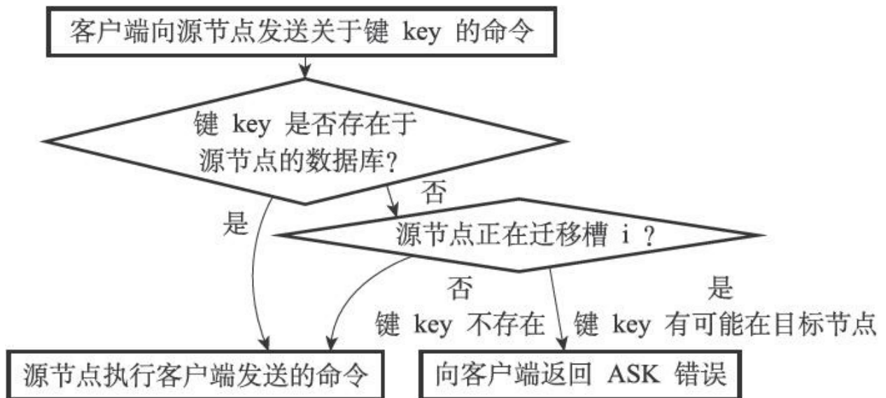
图17-26 判断是否发送ASK错误的过程
