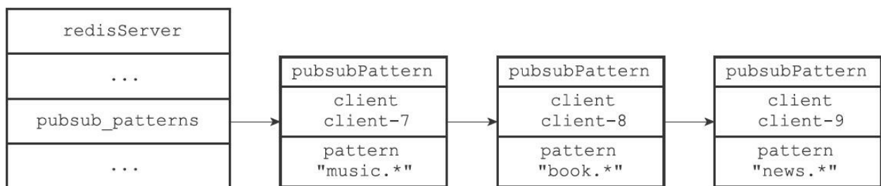
图18-11 pubsub_patterns链表示例
