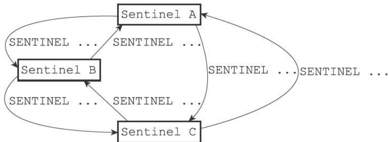
图16-21 Sentinel再次向其他Sentinel发送命令
