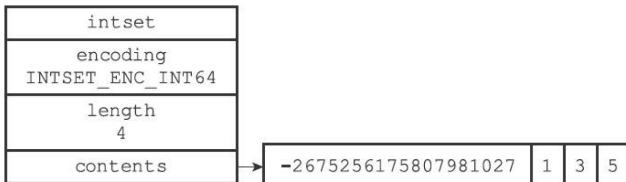
图6-2 一个包含四个int64_t类型整数值的整数集合
