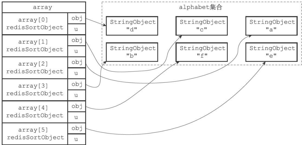
图21-15 将obj指针指向集合的各个元素
