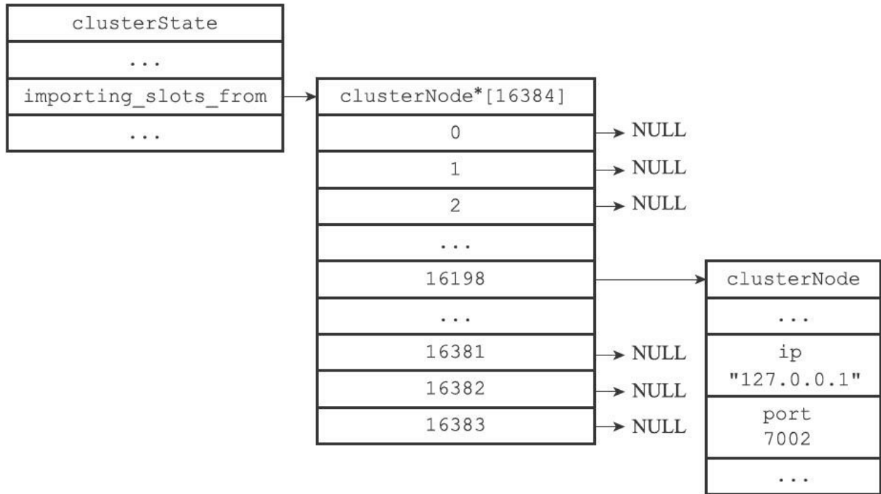
图17-27 节点7003的importing_slots_from数组
