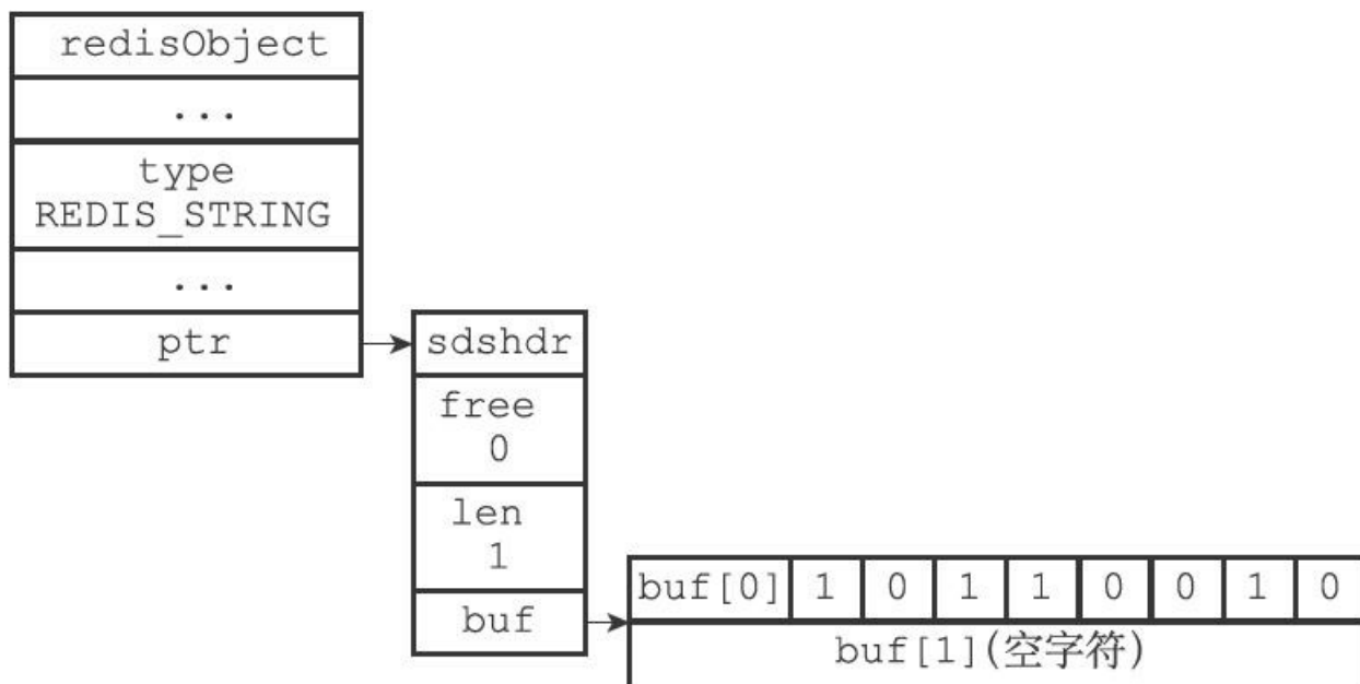
图22-2 一字节长的位数组的SDS表示
