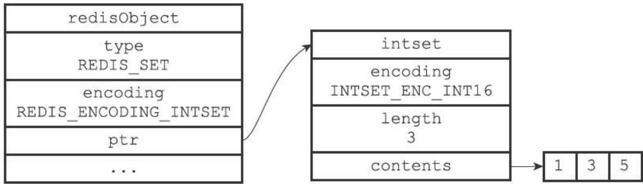
图8-12 intset编码的numbers集合对象
