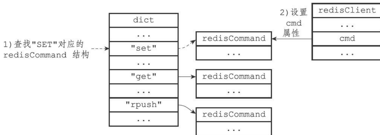
图13-7 查找命令并设置cmd属性
