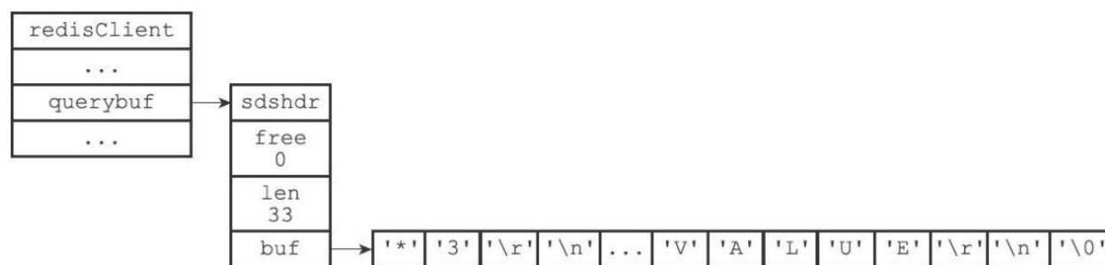
图14-2 客户端状态中的命令请求
