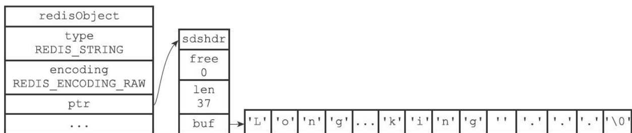
图8-2 raw编码的字符串对象
