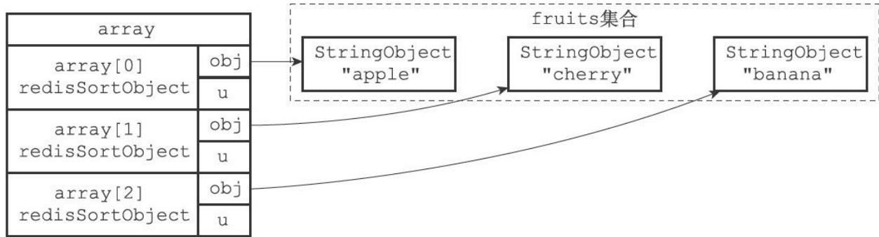
图21-12 将obj指针指向集合的各个元素
