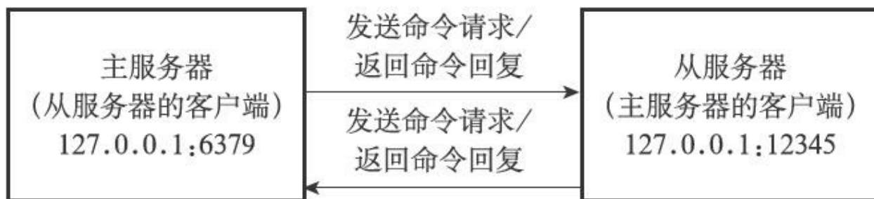
图15-22 主从服务器之间互为客户端
