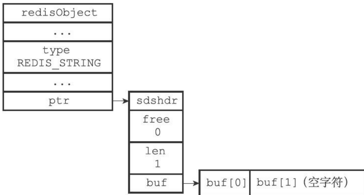
图22-1 SDS表示的位数组
