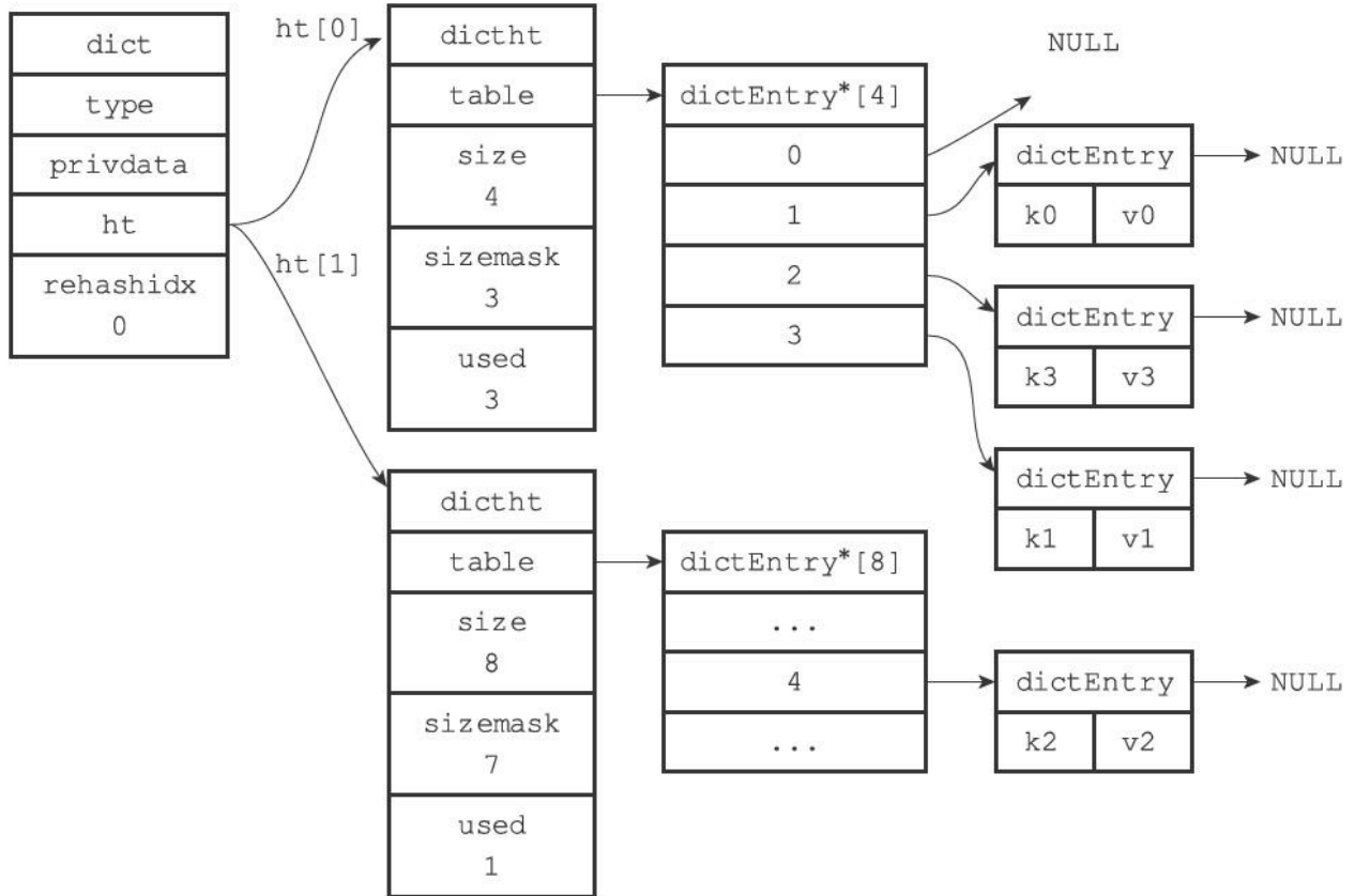
图4-13 rehash索引0上的键值对
