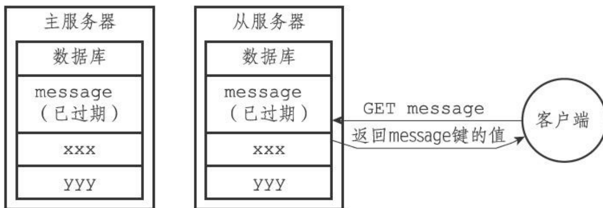
图9-18 主从服务器删除过期键 (2)
