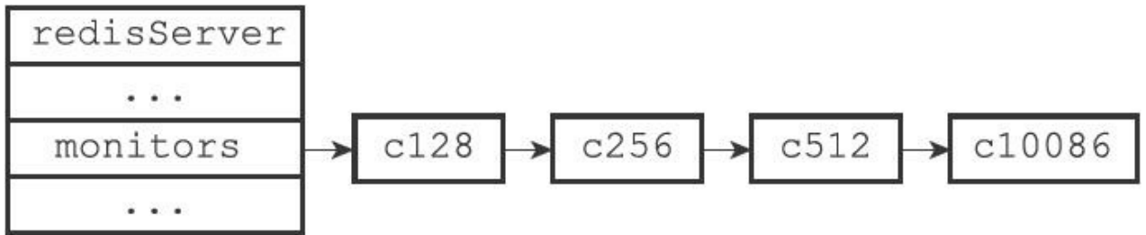
图24-3 客户端c10086执行MONITOR命令之后的monitors链表
