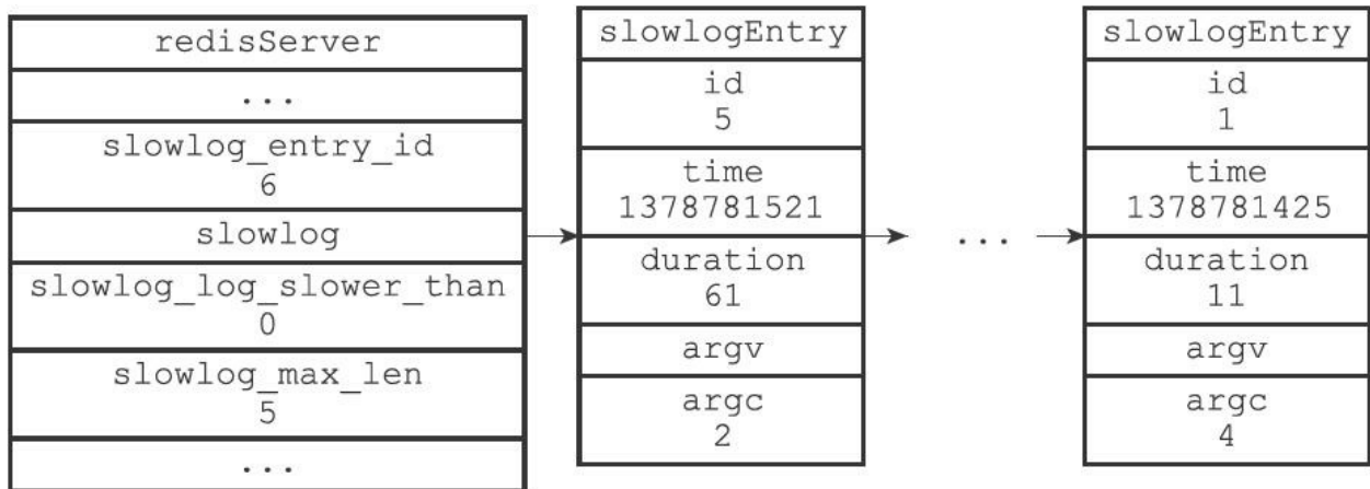
图23-2 redisServer结构示例
