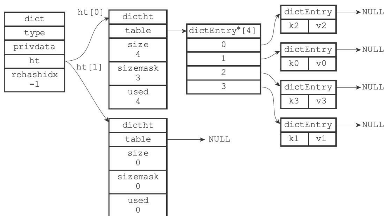
图4-8 执行rehash之前的字典
