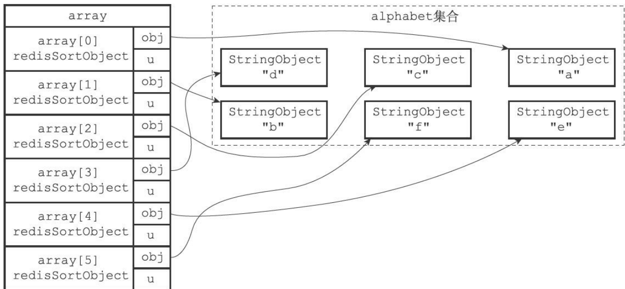
图21-16 排序后的数组
