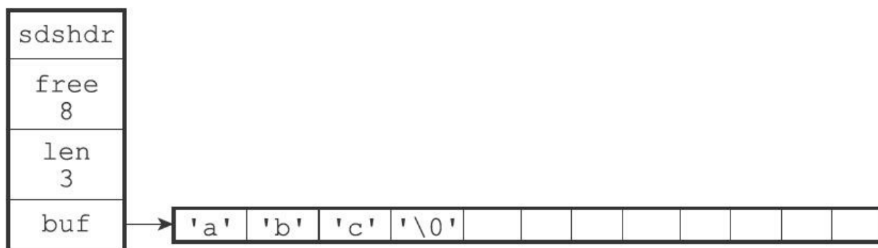
图2-15 执行sdstrim之后的SDS
