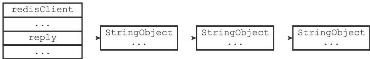
图13-9 可变大小缓冲区示例
