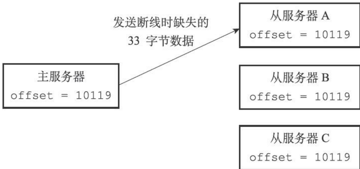
图15-11 主服务器向从服务器发送缺失的数据
