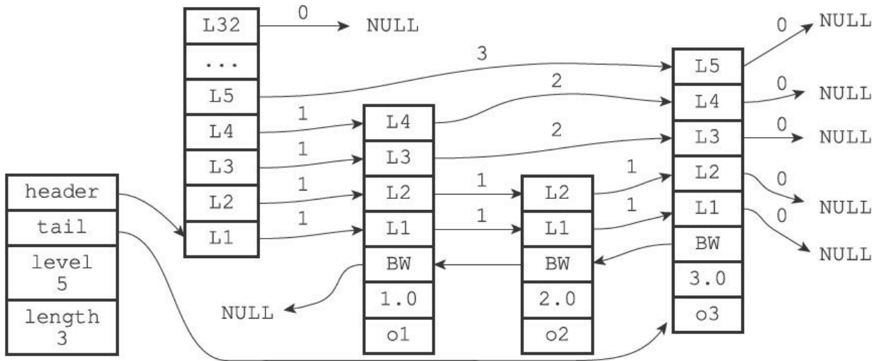
图5-9 带有zskiplist结构的跳跃表
