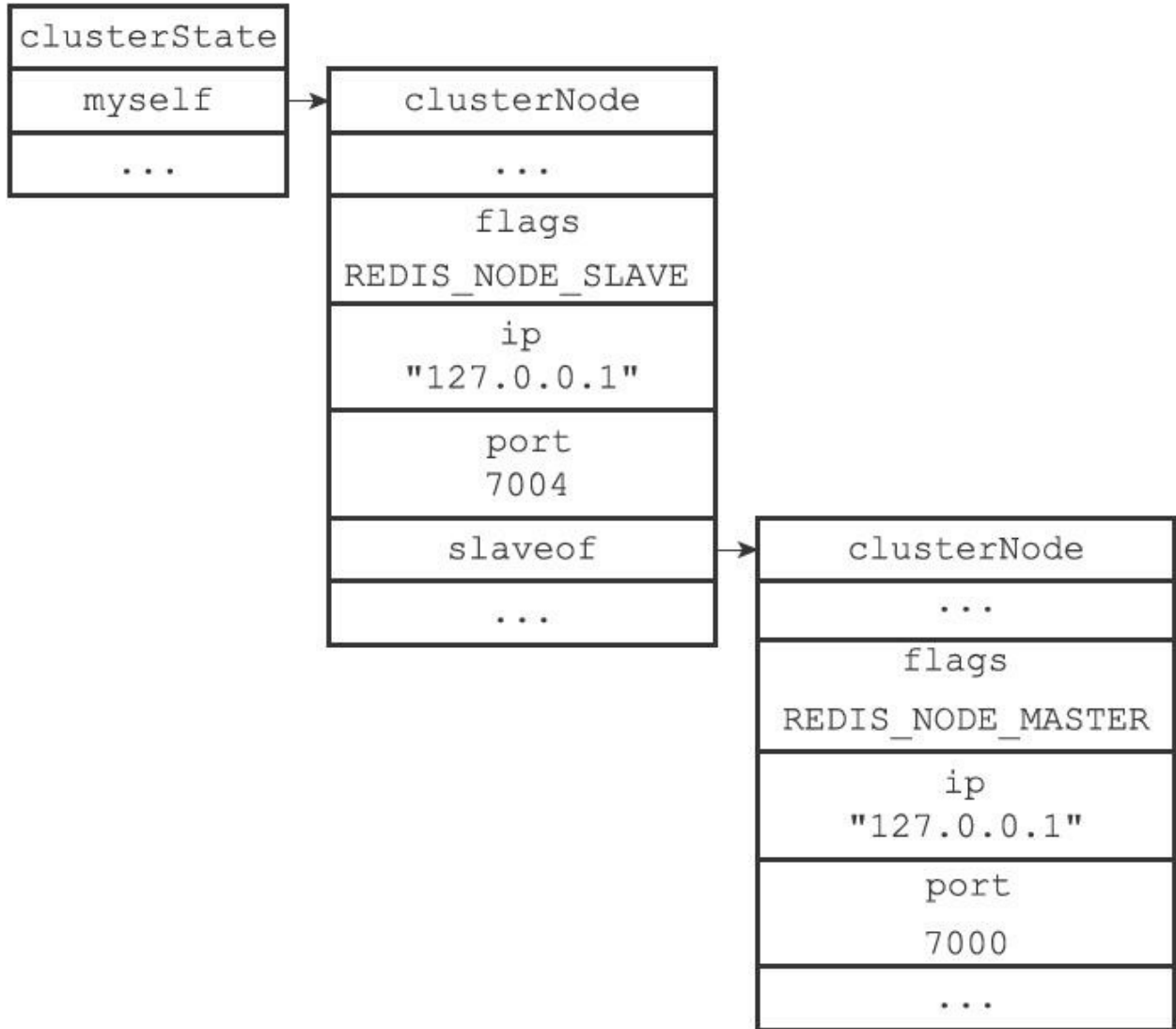
图17-35 节点7004的clusterState结构
