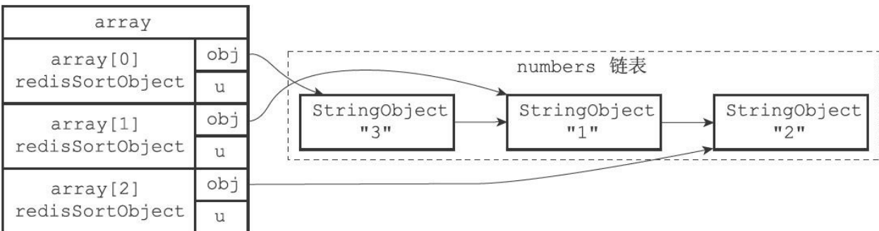
图21-2 将obj指针指向列表的各个项
