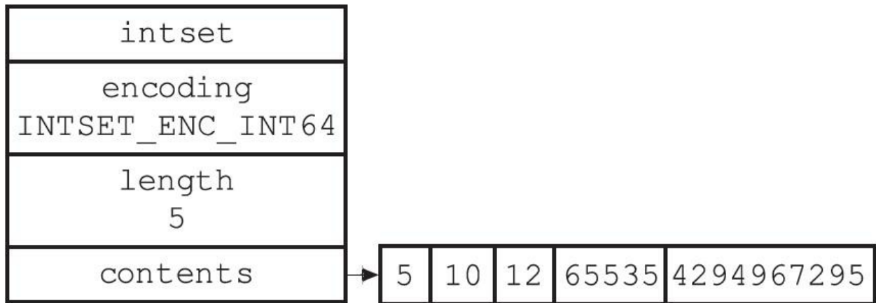
图6-11 数组编码为 INTSET_ENC_INT64 的整数集合
