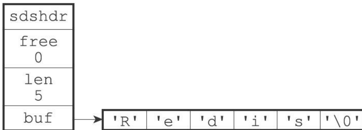
图2-5 5字节长的SDS
