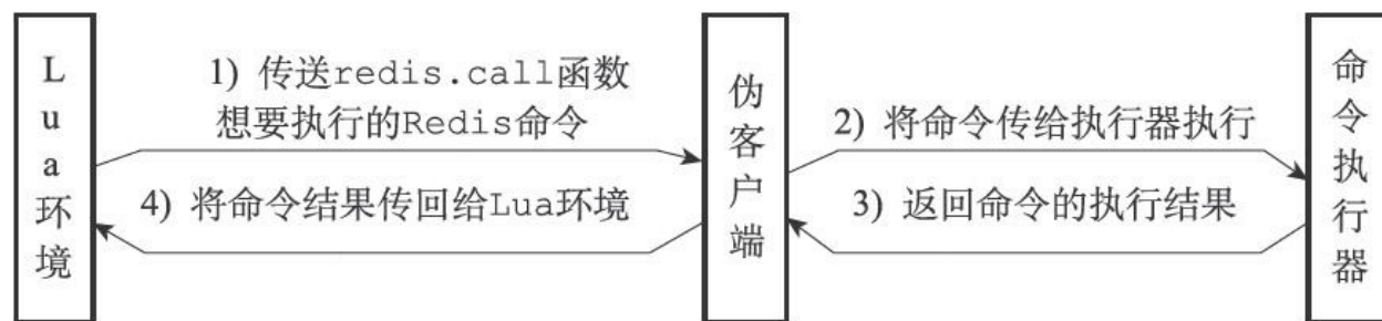
图20-2 Lua脚本执行Redis命令时的通信步骤
