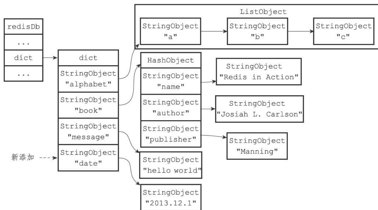
图9-5 添加date键之后的键空间
