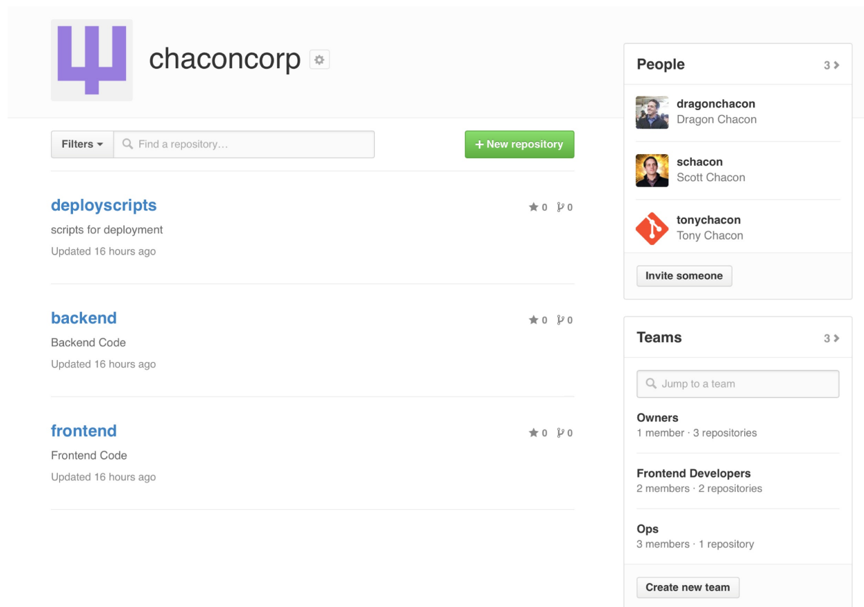
Figure 6-46. 组织页面
