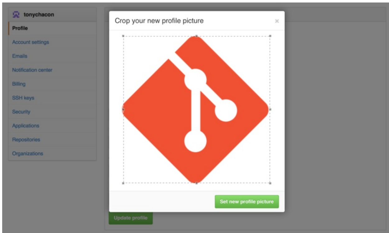
Figure 6-5. 裁剪头像
