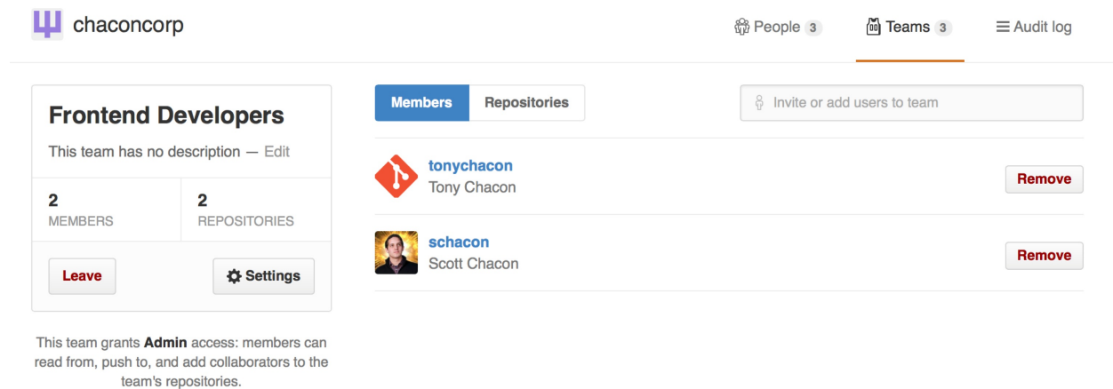
Figure 6-47. 团队页面
